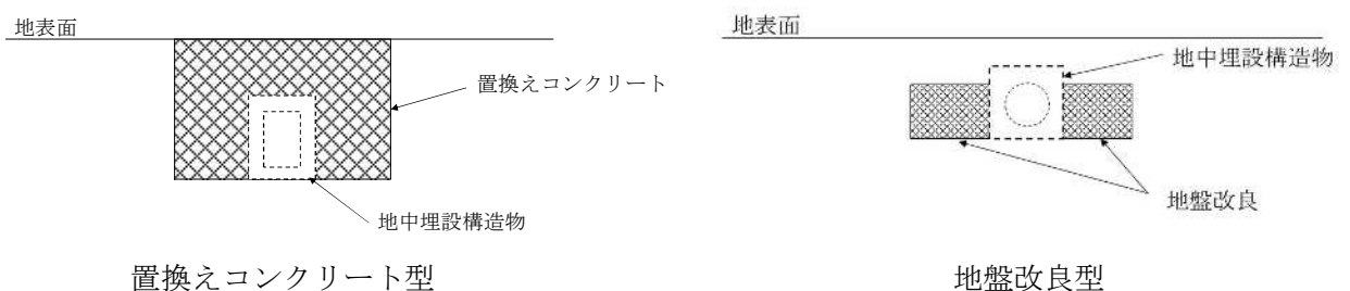
図9-7 浮上り対策
