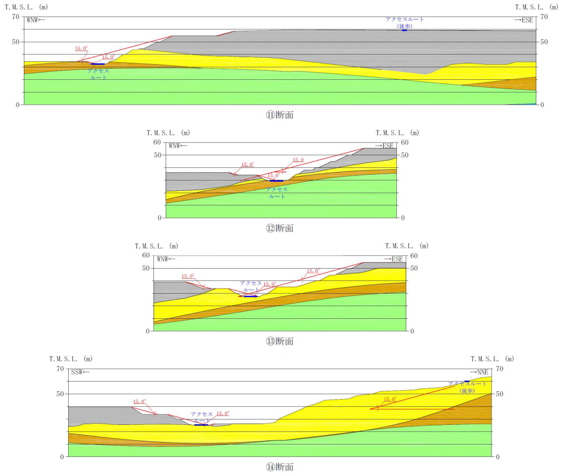
図 3-9 影響評価断面位置における斜面の崩壊形状を想定した結果 (2/3)
