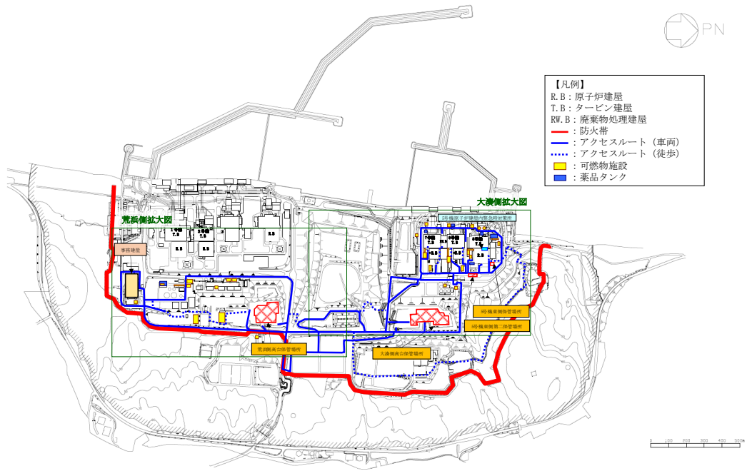
(全体図)
