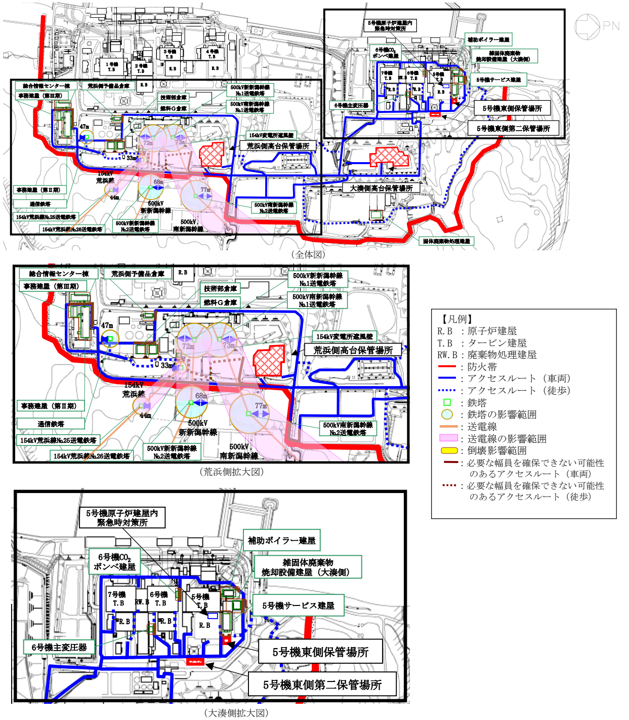
図 3-2 倒壊時にアクセスルートに影響を及ぼす周辺構造物配置図
