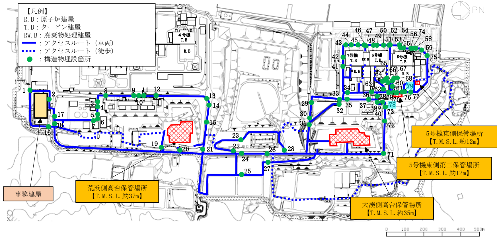
図 3-11 地中埋設構造物と埋戻部等との境界部における不等沈下の評価位置
