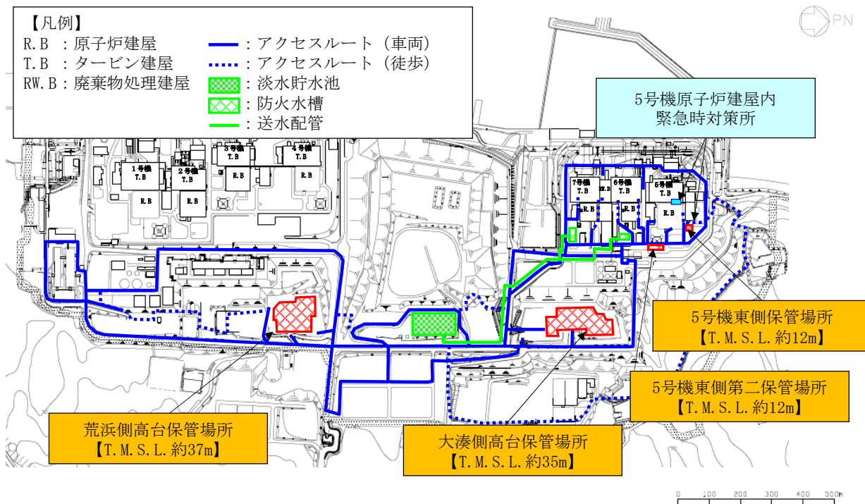
図3-18 淡水貯水池及び送水配管の位置図
