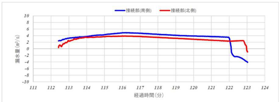
図5 漏水量の経時変化図（基準津波2）
