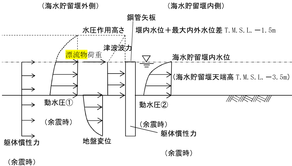
図 2.3-3-5 荷重作用図（鋼管矢板 重畳時 2）
