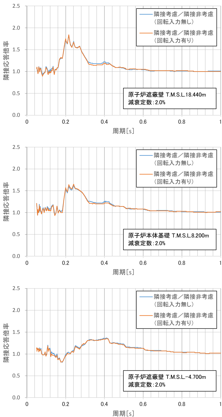
図添 6-1 回転入力の影響 (床応答スペクトル)
