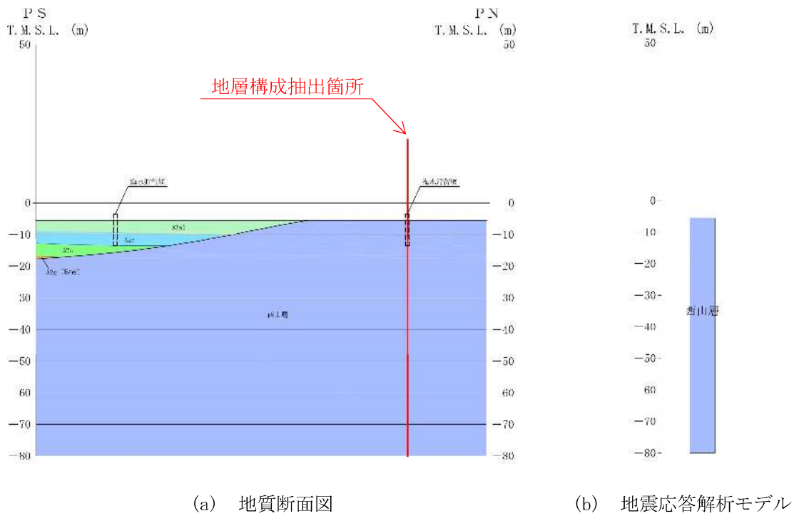
図 3-2 (1) 評価対象 A-A 断面図 (断面①)
