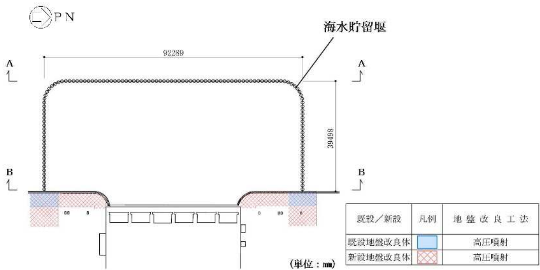
図 3-1 海水貯留堰の評価対象断面位置図
