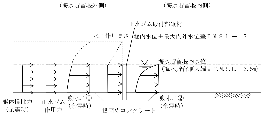
図 3-8 荷重作用図 (止水ゴム取付部鋼材 重畳時 2)
