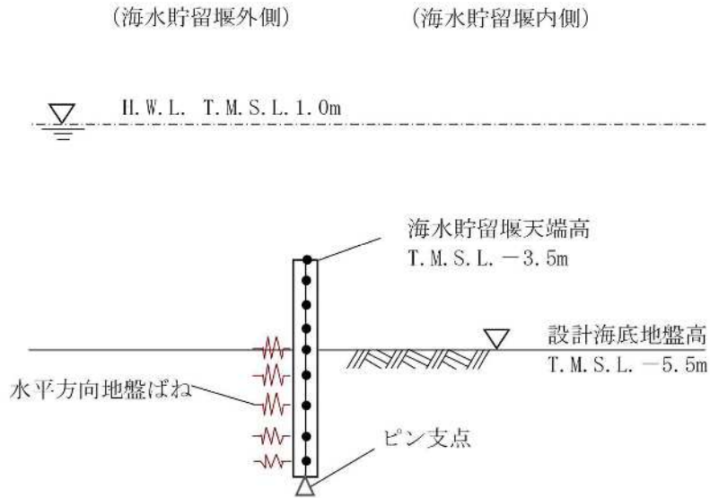
図 3-9 解析モデル
