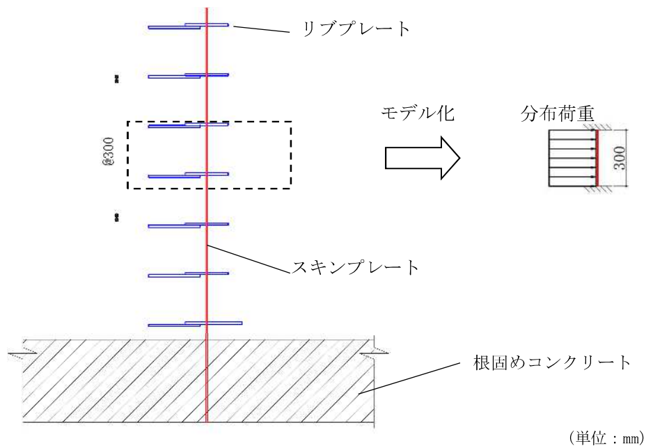
図 3-11 スキンプレート照査モデル図
