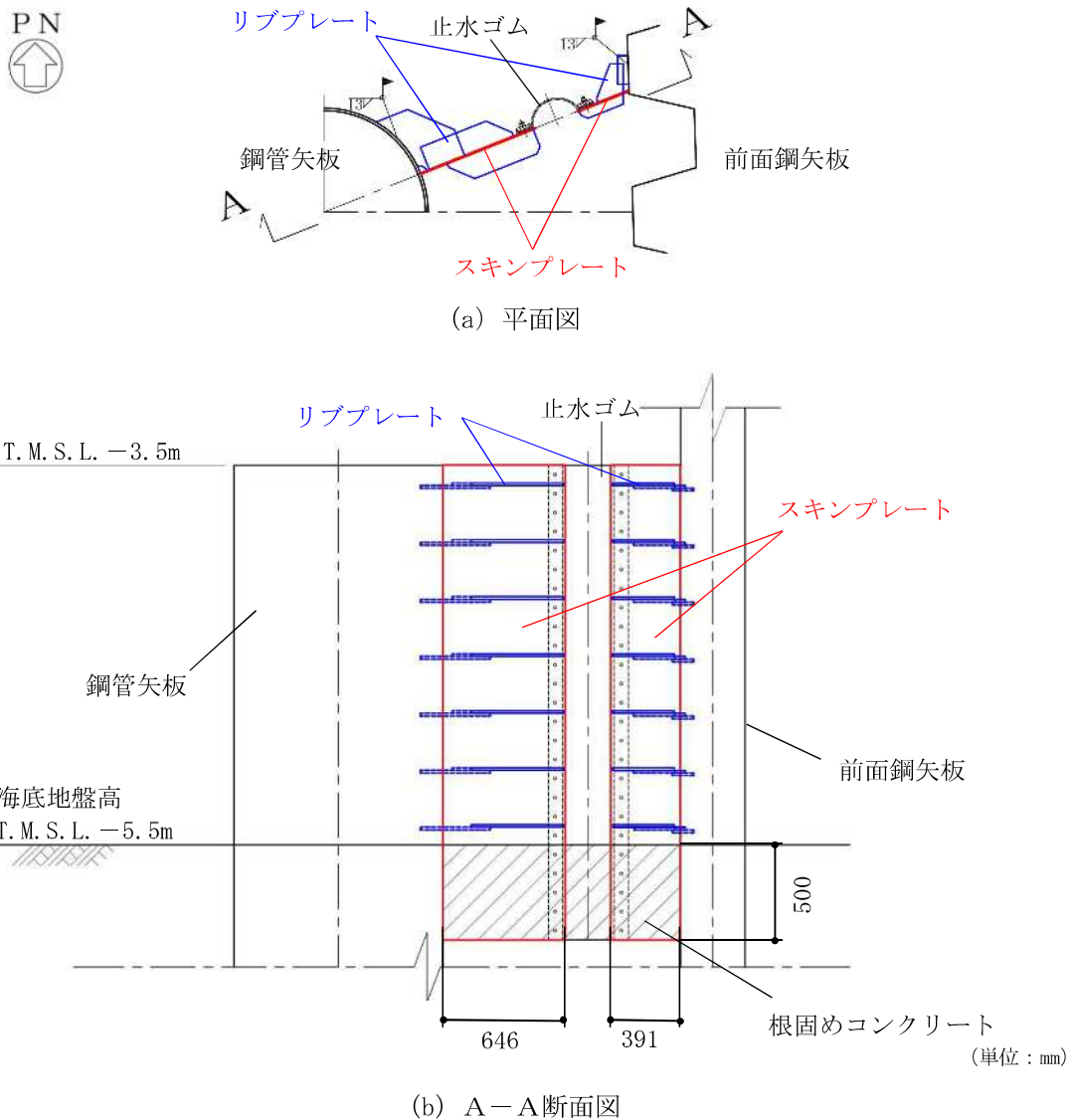
図 3-10 (1) 詳細構造図 (南側)
