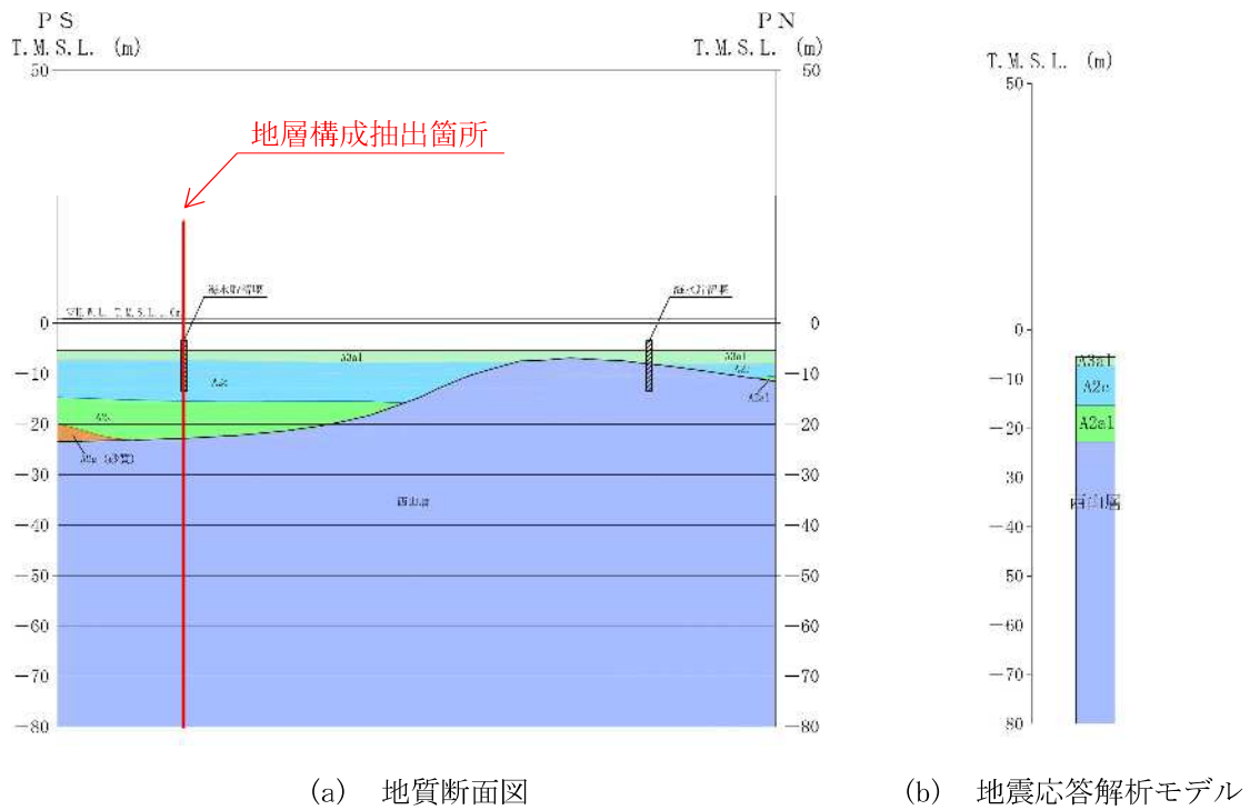
図 3-2 (2) 評価対象 B-B 断面図 (断面②)
