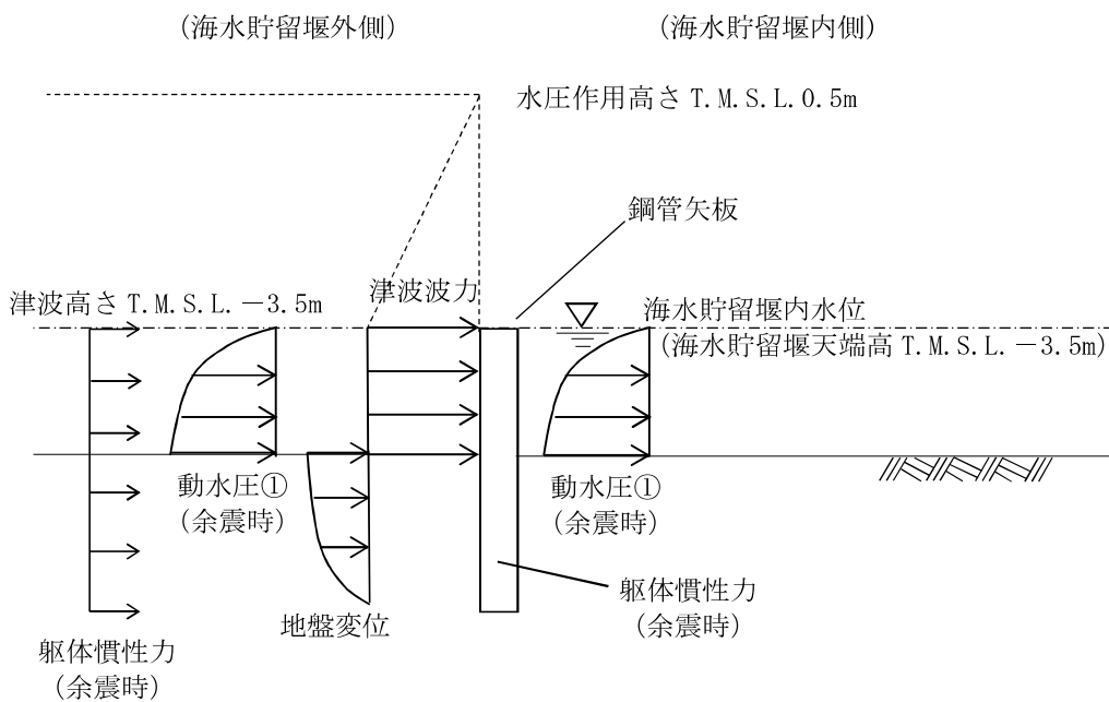
図 3-4 荷重作用図 (鋼管矢板 重畳時 1)
