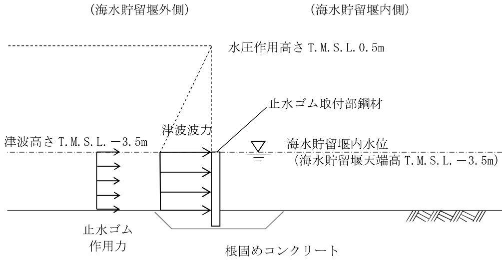
図 3-6 荷重作用図 (止水ゴム取付部鋼材 津波時)
