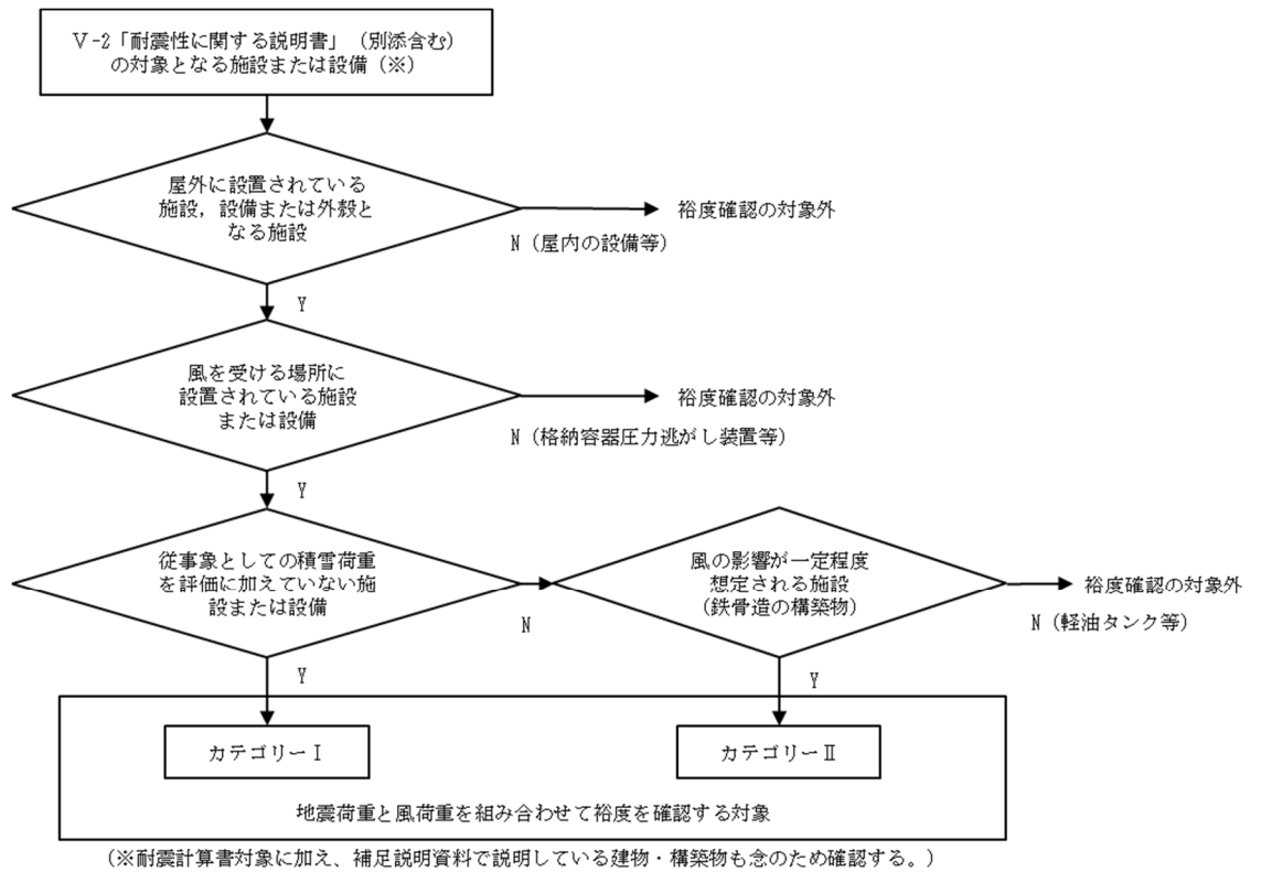
図1 地震荷重と風荷重を組み合わせる対象選定フロー
