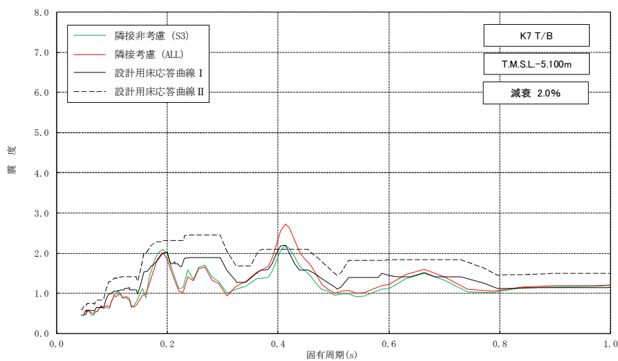
図添 1-3 床応答スペクトルの比較 (7号機タービン建屋, 水平方向, 減衰 2.0%) (3/3)
