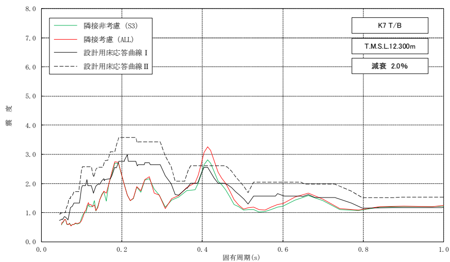
図添 1-3 床応答スペクトルの比較 (7号機タービン建屋, 水平方向, 減衰 2.0%) (2/3)
