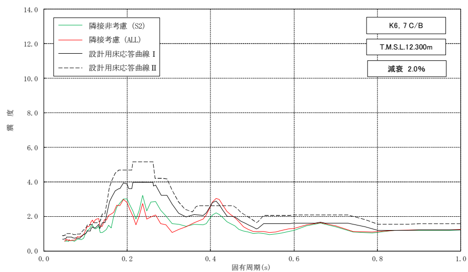
図添 1-2 床応答スペクトルの比較 (コントロール建屋, 水平方向, 減衰 2.0%) (1/2)
