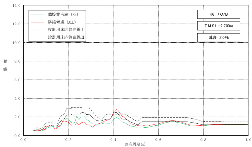
図添 1-2 床応答スペクトルの比較 (コントロール建屋, 水平方向, 減衰 2.0%) (2/2)
