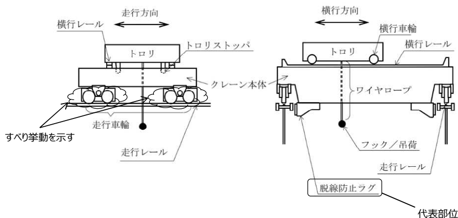
図2-4 原子炉建屋クレーンの構造図
