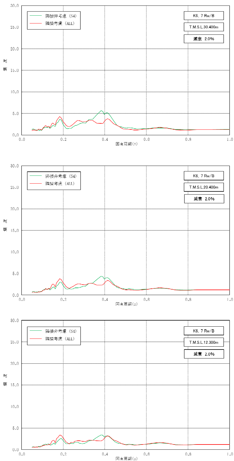
図添 1-4 床応答スペクトルの比較（廃棄物処理建屋，水平方向，減衰 2.0%）（2/3）
