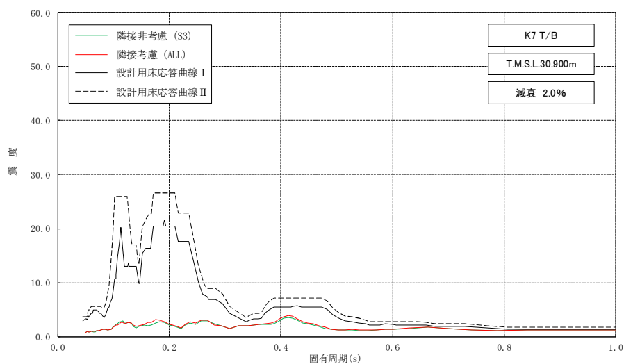
図添 1-3 床応答スペクトルの比較 (7号機タービン建屋, 水平方向, 減衰 2.0%) (1/3)
