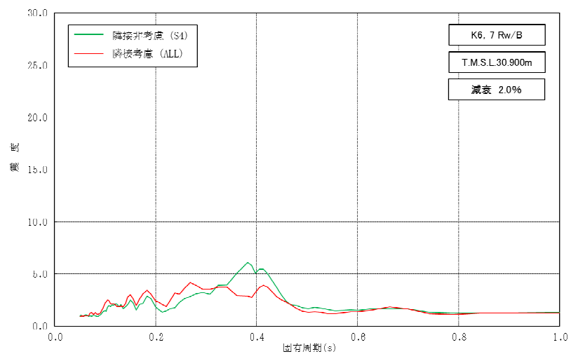
図添 1-4 床応答スペクトルの比較（廃棄物処理建屋，水平方向，減衰 2.0%）（1/3）
