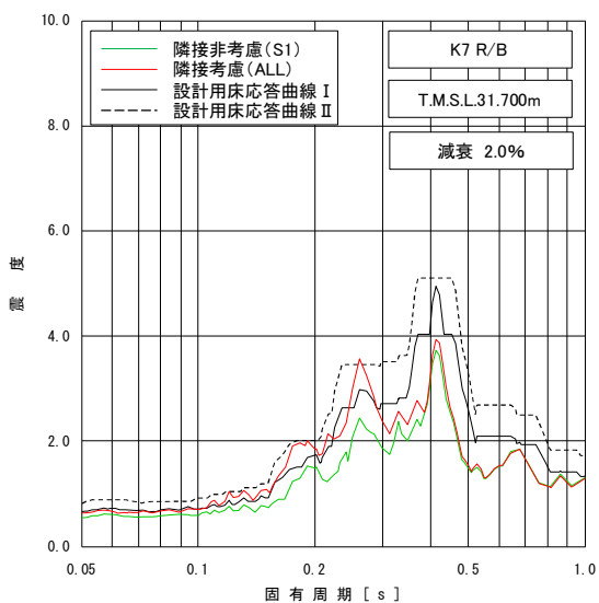
図添 1-1 床応答スペクトルの比較 (7号機原子炉建屋, 水平方向, 減衰 2.0%) (1/3) 別紙 4-12
