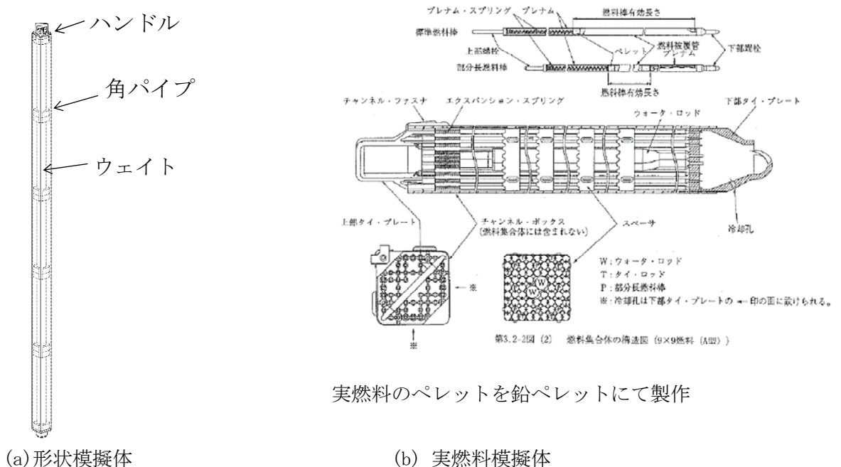
第6図 模擬燃料集合体の内部構造
