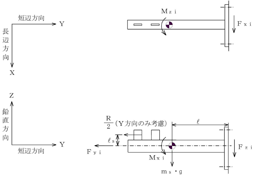
図5-3 荷重状態
