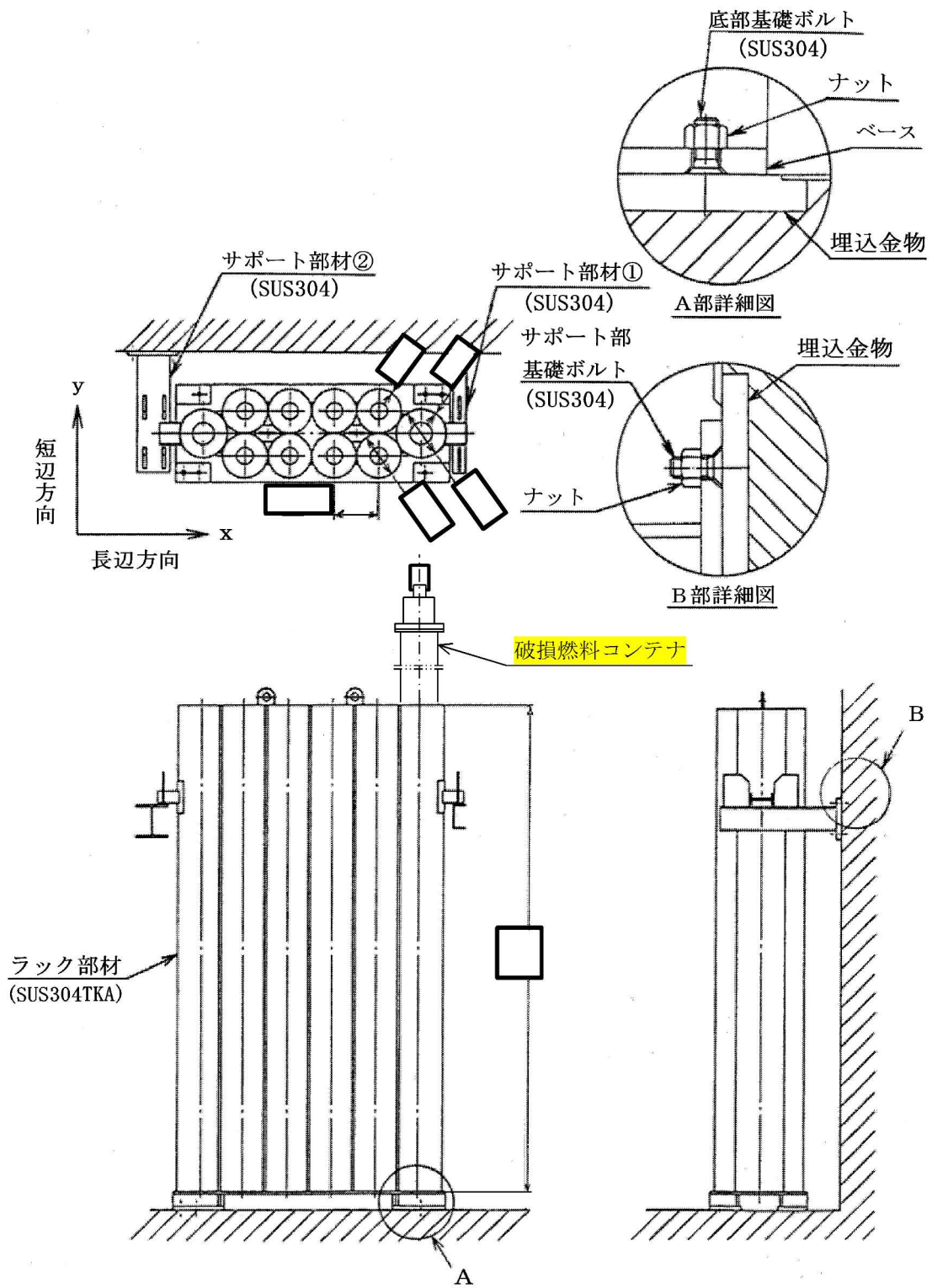
図 3-1 構造概要図 (単位 : mm)
