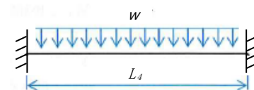
図 3-5 両端固定梁
