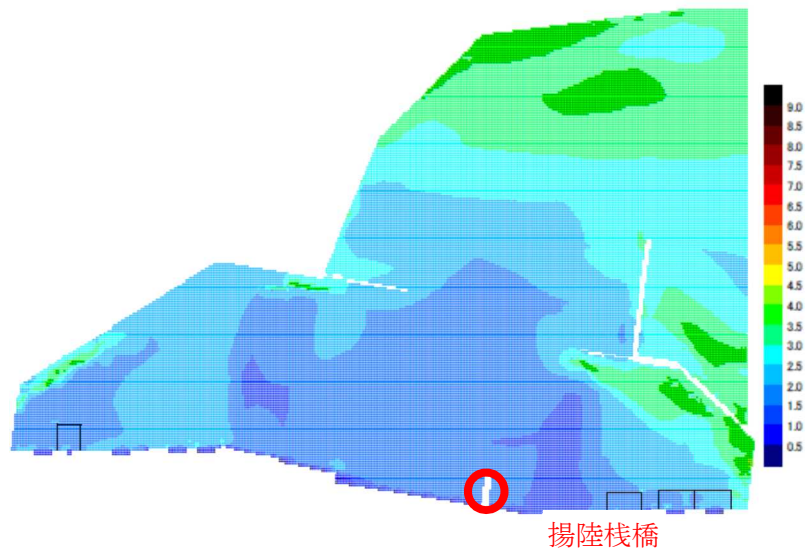
第10図 基準津波3 防波堤なし 12hrs 最大流速コンター図
