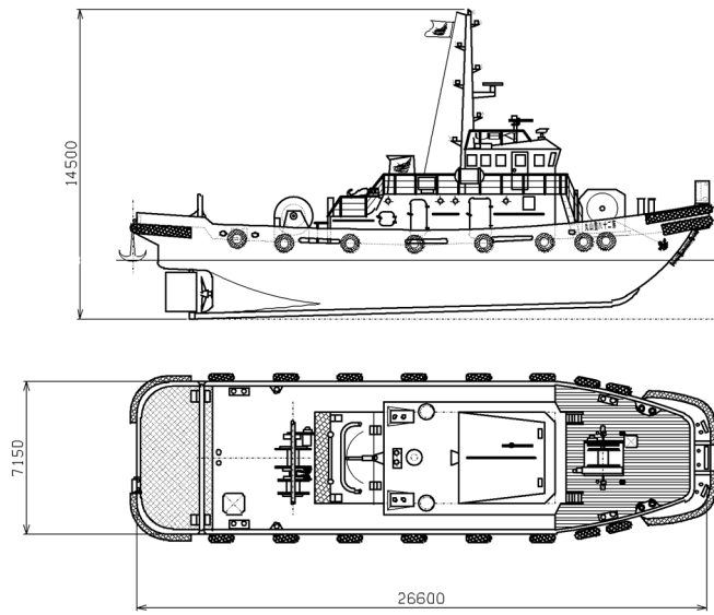
第2図 曳船の外形図
