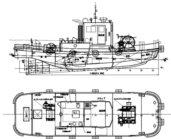
第3図 揚錨船の外形図
