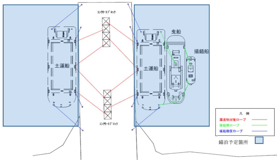
第4図 土運船 揚陸栈橋への錨泊状態 (例)
