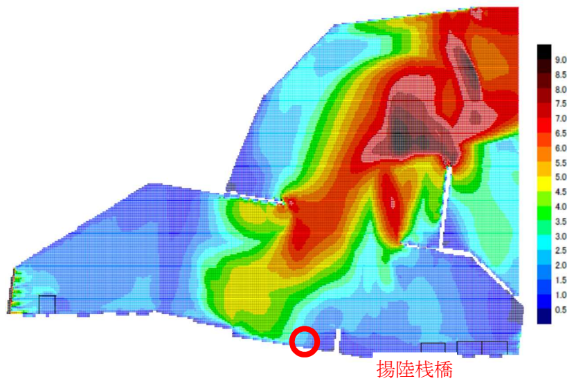
第 7 図 基準津波 3 防波堤あり 12hrs 最大流速コンター図
