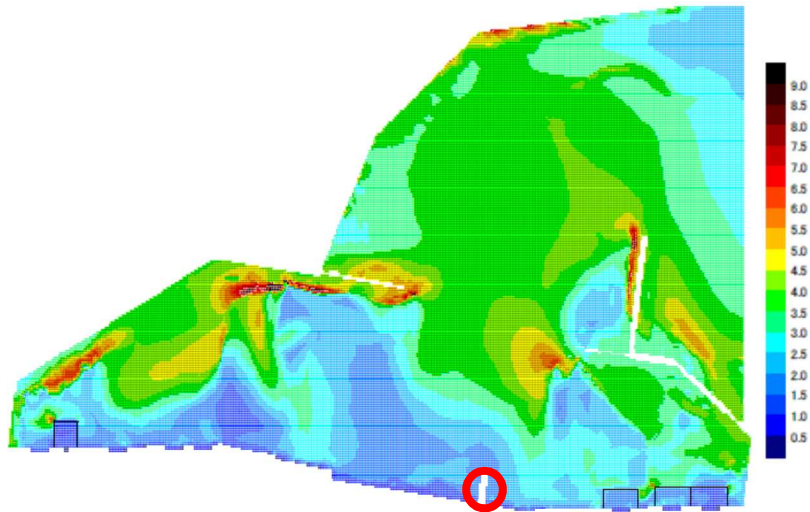
第9図 基準津波2 防波堤なし 12hrs 最大流速コンター図
