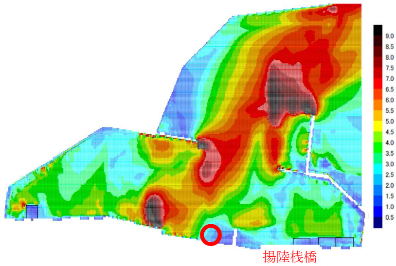
第 6 図 基準津波 2 防波堤あり 12hrs 最大流速コンター図
