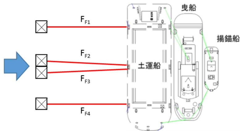
第 13 図 作用する力の関係イメージ（平面）
