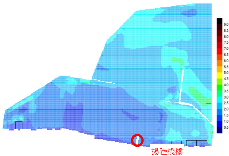
第 8 図 基準津内 1 防波堤なし 12hrs 最大流速コンター図
