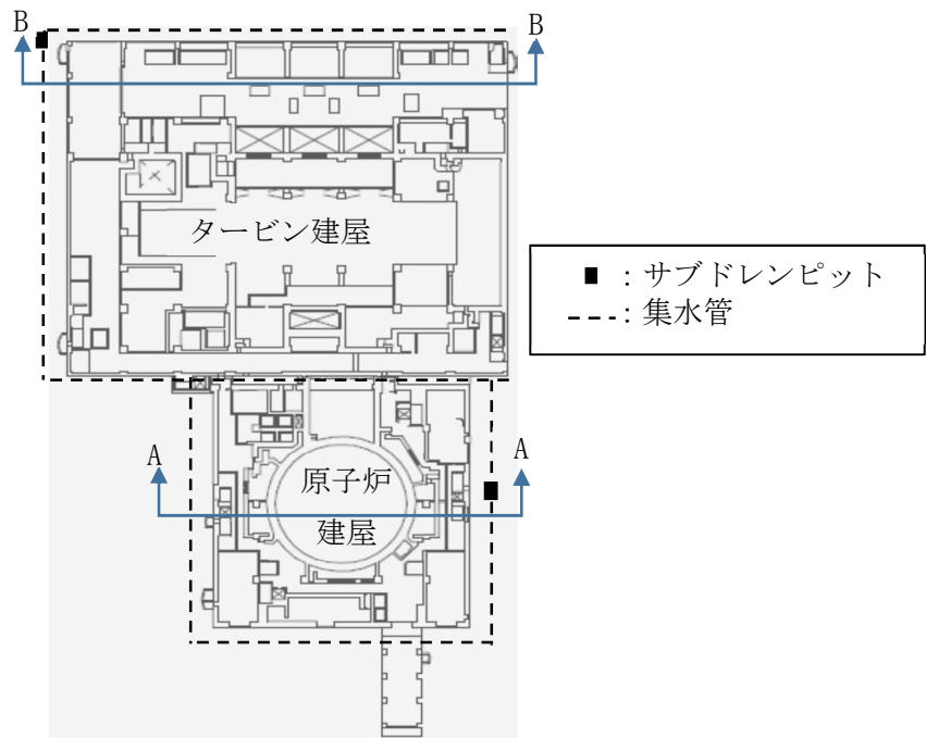
(1) サブドレンピット，集水管の配置
