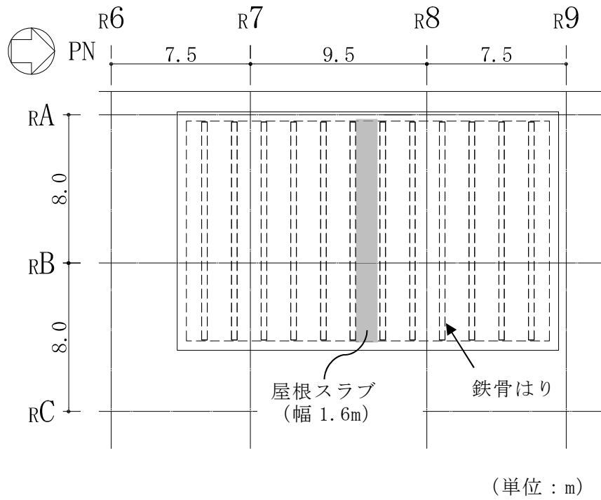
(c) 緊急時対策所 (対策本部) 屋根スラブ
