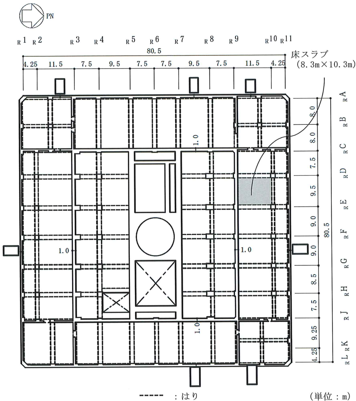
(a) 緊急時対策所 床スラブ
