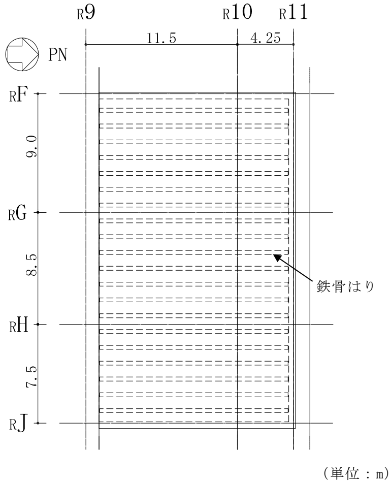
(d) 緊急時対策所 (待機場所) 屋根スラブ
