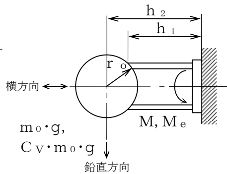
図4-2 鉛直方向荷重による胴板の脚付け根部のモーメント
