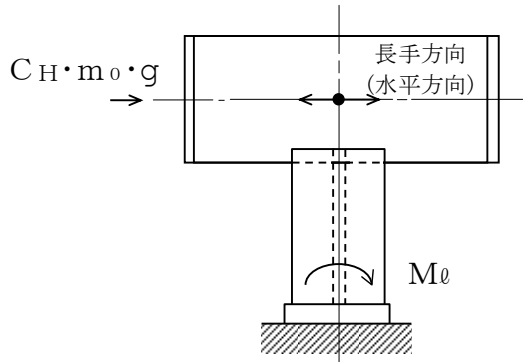
図4-1 長手方向荷重による胴板の脚付け根部のモーメント
