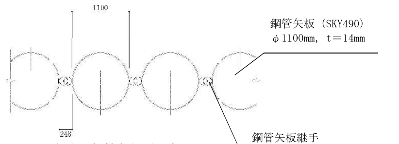
(d) 鋼管矢板継手部平面図
