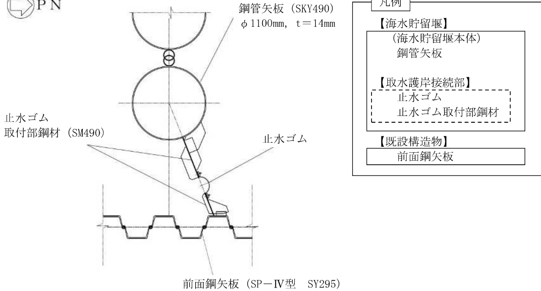
図 2.3-2-2(2) 海水貯留堰の平面図 (A部拡大)
