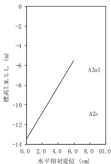
図 2.3-5-7 地盤変位分布図（断面②）
