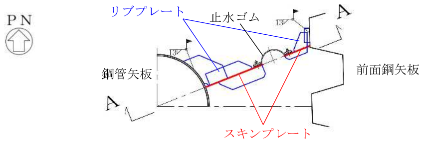
(a) 平面図
