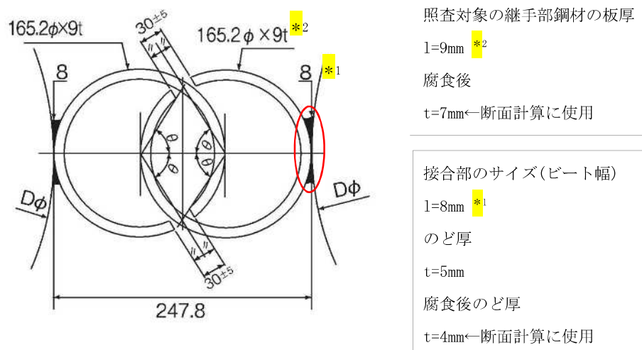
図 3 継手部の仕様
