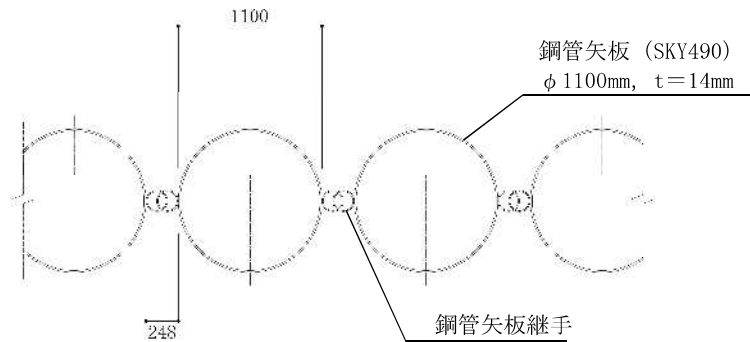
(c) 鋼管矢板継手部平面図
