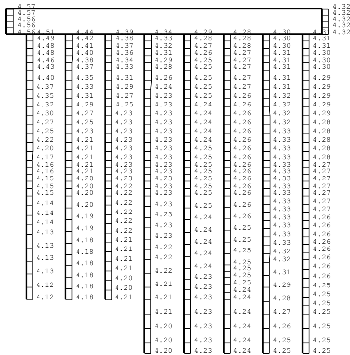
(b) Ss-3一十, 鉛直
