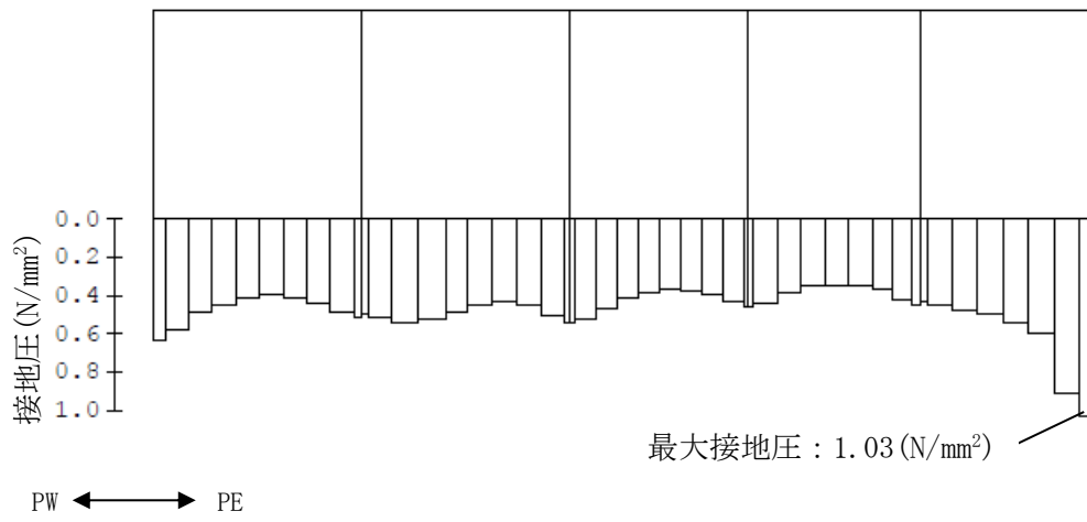
図 3-10 (1) 補機冷却用海水取水路の最大接地圧分布図 (南側, 解析ケース①, Ss-1--)
