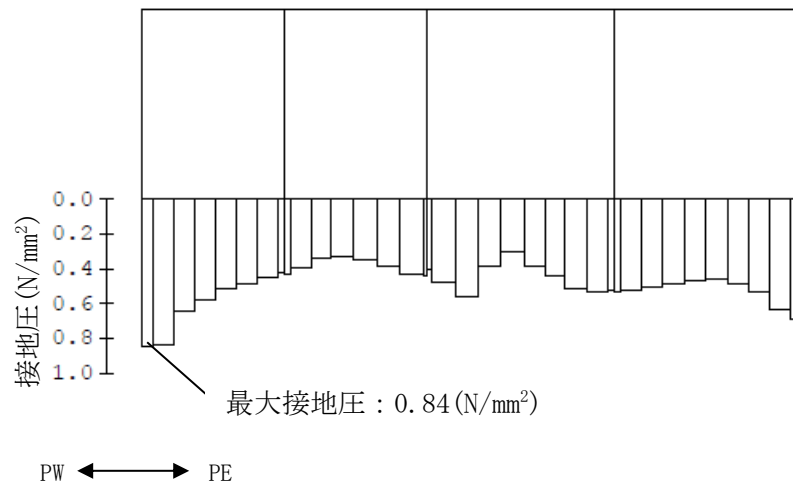
図 3-10 (2) 補機冷却用海水取水路の最大接地圧分布図 (北側, 解析ケース②, Ss-1+-)
