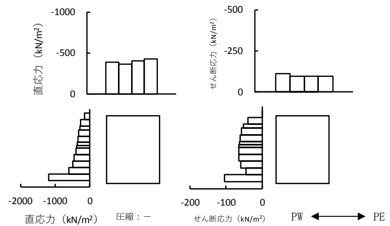
(c) B-B断面の作用荷重分布 (北妻壁)
