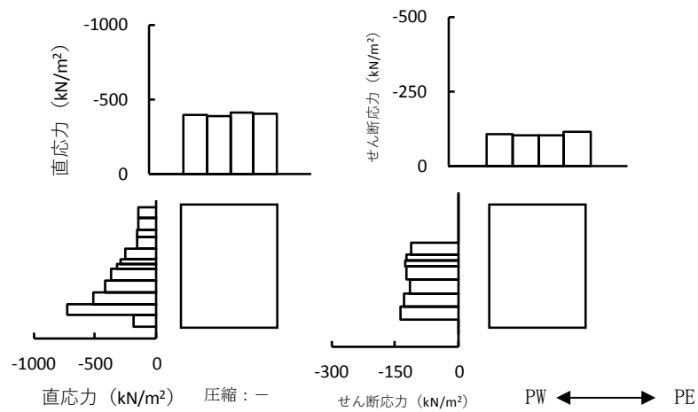
(b) B-B断面の作用荷重分布 (南妻壁)
