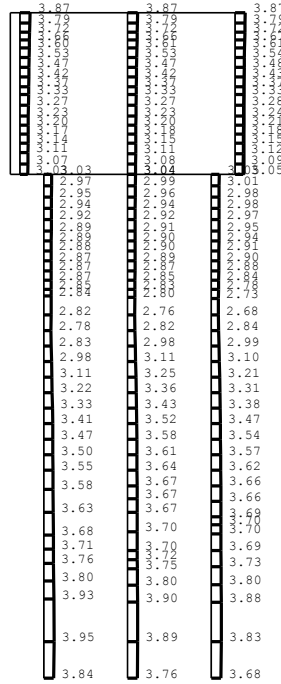
(a) Ss-2NS, 水平
