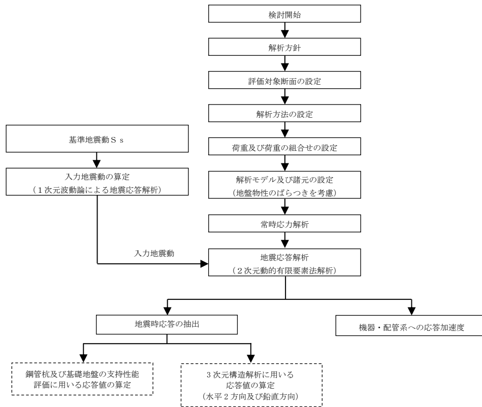
図 2-4 常設代替交流電源設備基礎の地震応答解析フロー
