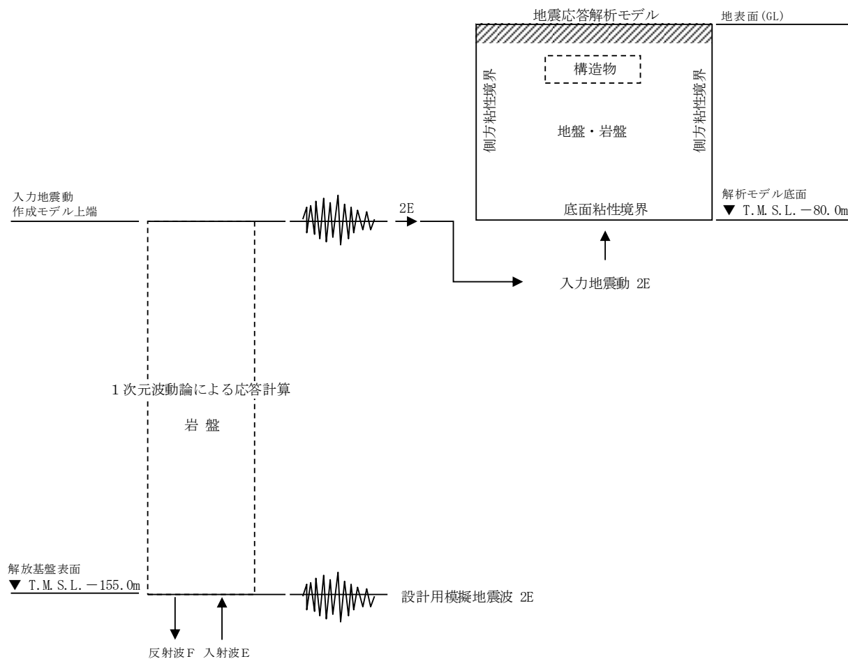
図 3-5 入力地震動算定の概念図
