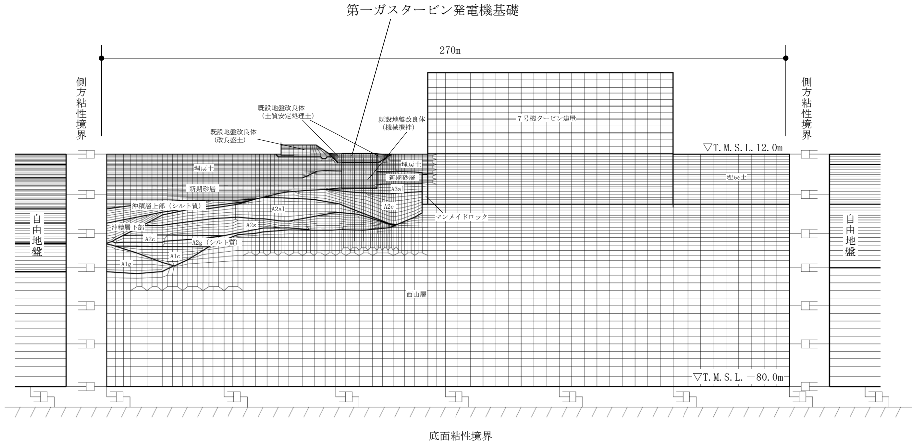
図 3-7 (1) 常設代替交流電源設備基礎の地震応答解析モデル (A-A断面)
