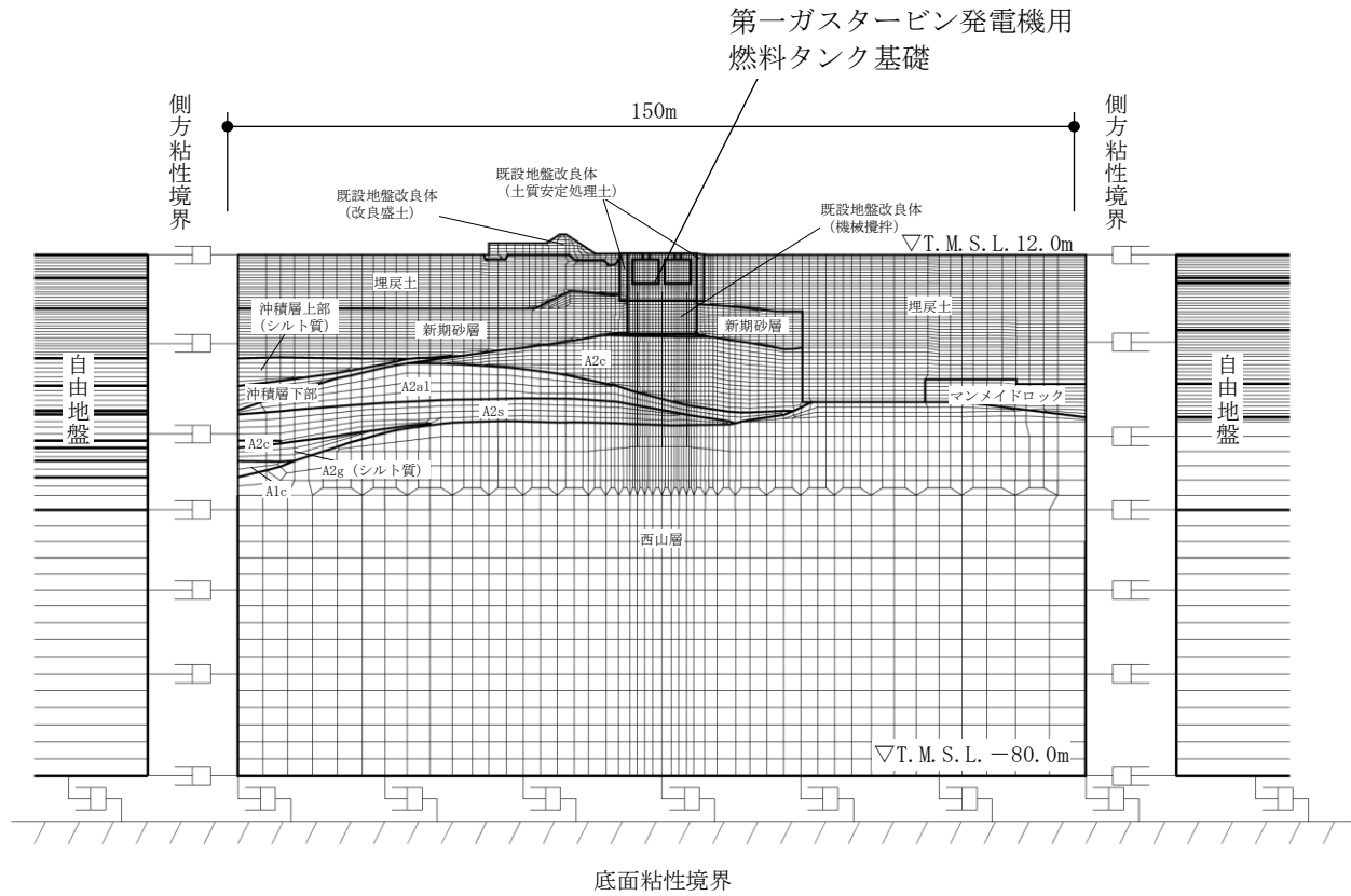
図 3-7 (2) 常設代替交流電源設備基礎の地震応答解析モデル (B-B断面)
