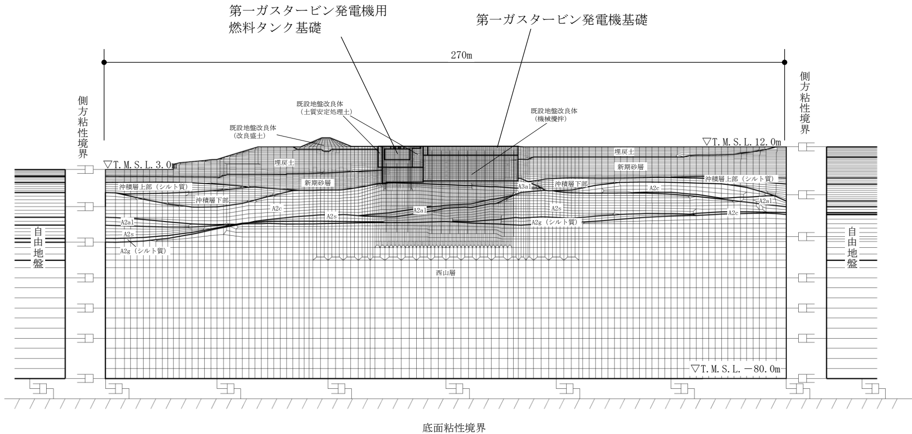
図 3-7 (3) 常設代替交流電源設備基礎の地震応答解析モデル (C-C断面)
