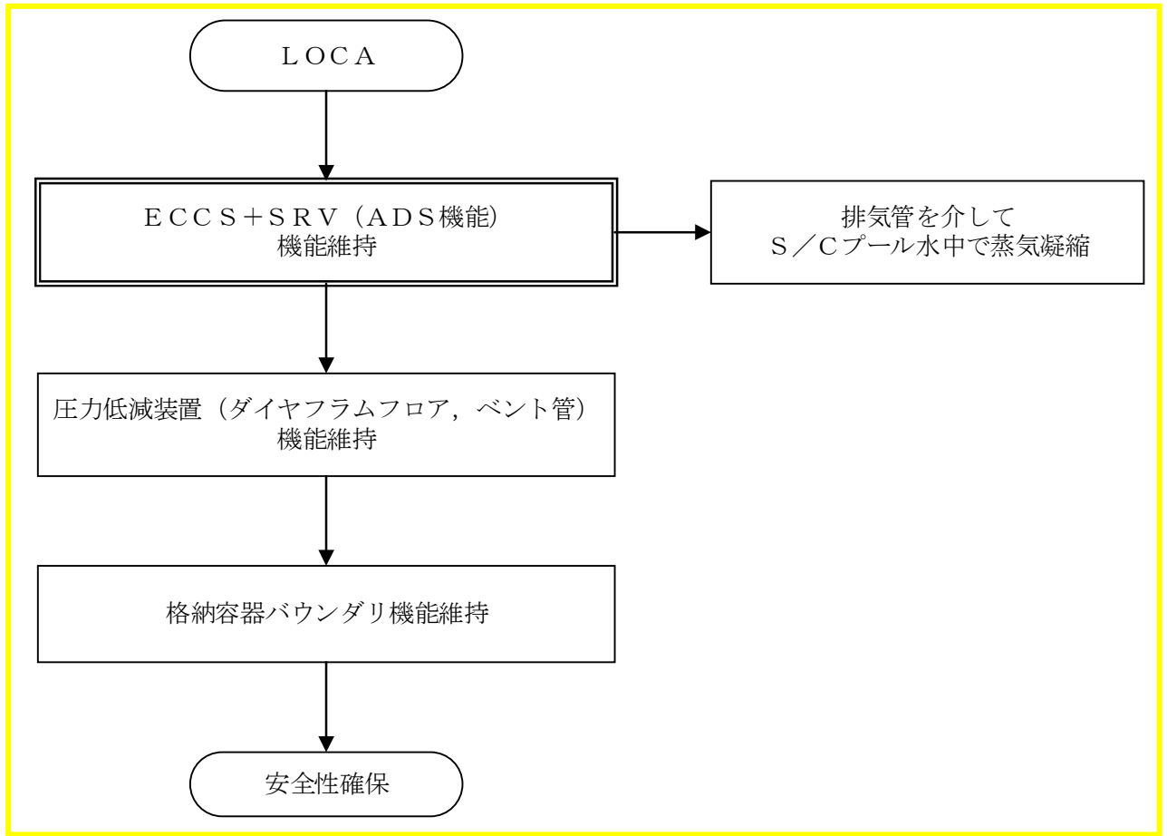
図2 LOCA後のプラントシーケンス
