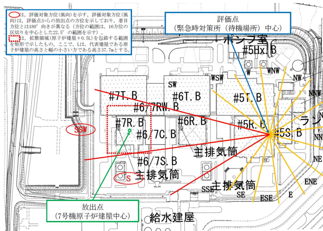
図4-3 評価対象とする風向 (4/4)
