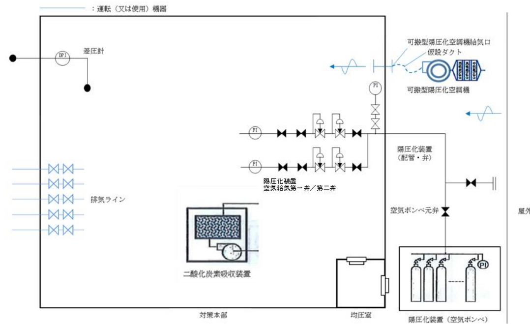
図3-3 緊急時対策所（対策本部）換気空調系 構成図 （放射性雲通過前及び通過後：可搬型陽圧化空調機（対策本部）による陽圧化）
