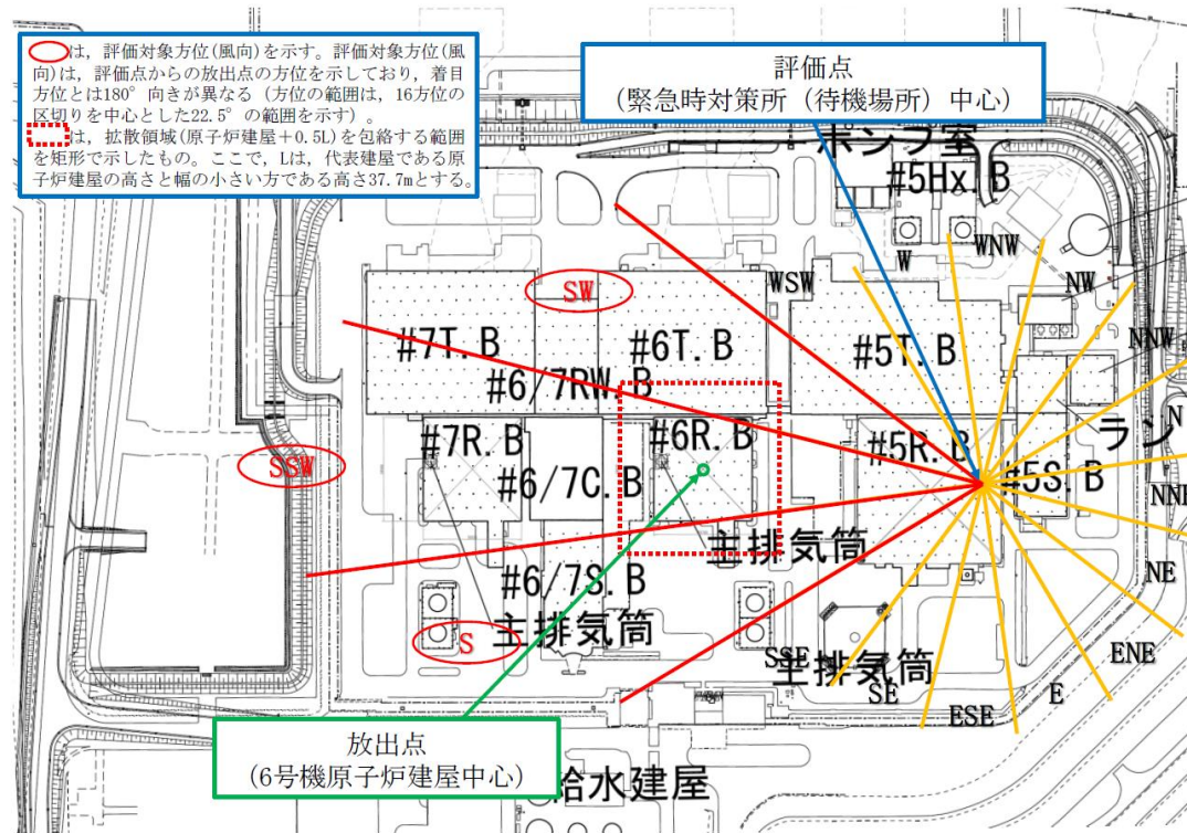
図4-3 評価対象とする風向 (3/4)
