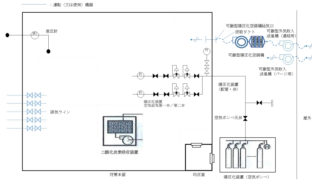
図3-5 緊急時対策所(対策本部)換気空調系構成図 (放射性雲通過直後に建屋内の放射性物質濃度が屋外より高い場合:可搬型外気取入送風機及び可搬型陽圧化空調機(対策本部)の連結運用による外気取り入れ陽圧化,並びに建屋内空気置換)
