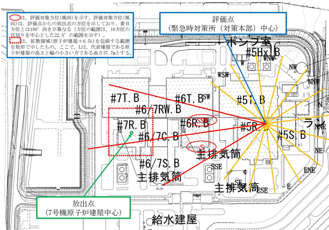
図4-3 評価対象とする風向 (2/4)
