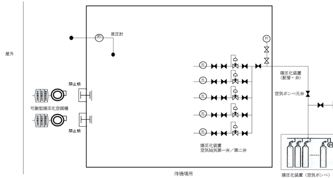
図 3-1 緊急時対策所（対策本部）換気空調系 構成図
