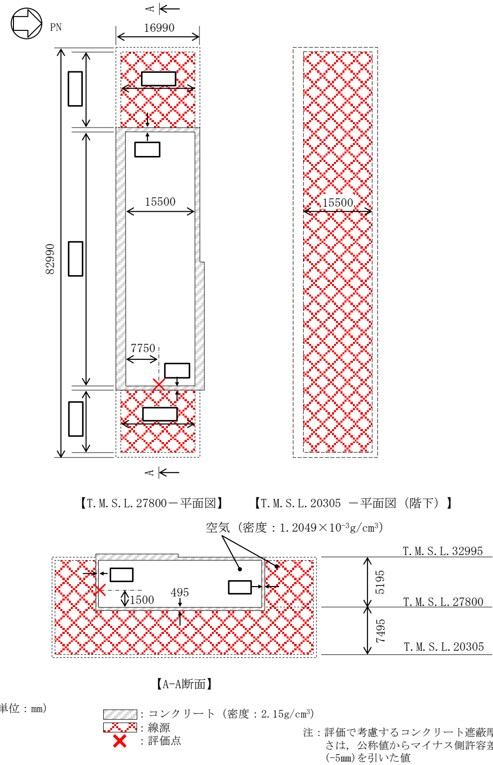
図4-13 隣接エリア内に取り込まれた放射性物質による被ばくの評価モデル図 (2/2) (緊急時対策所 (待機場所))
