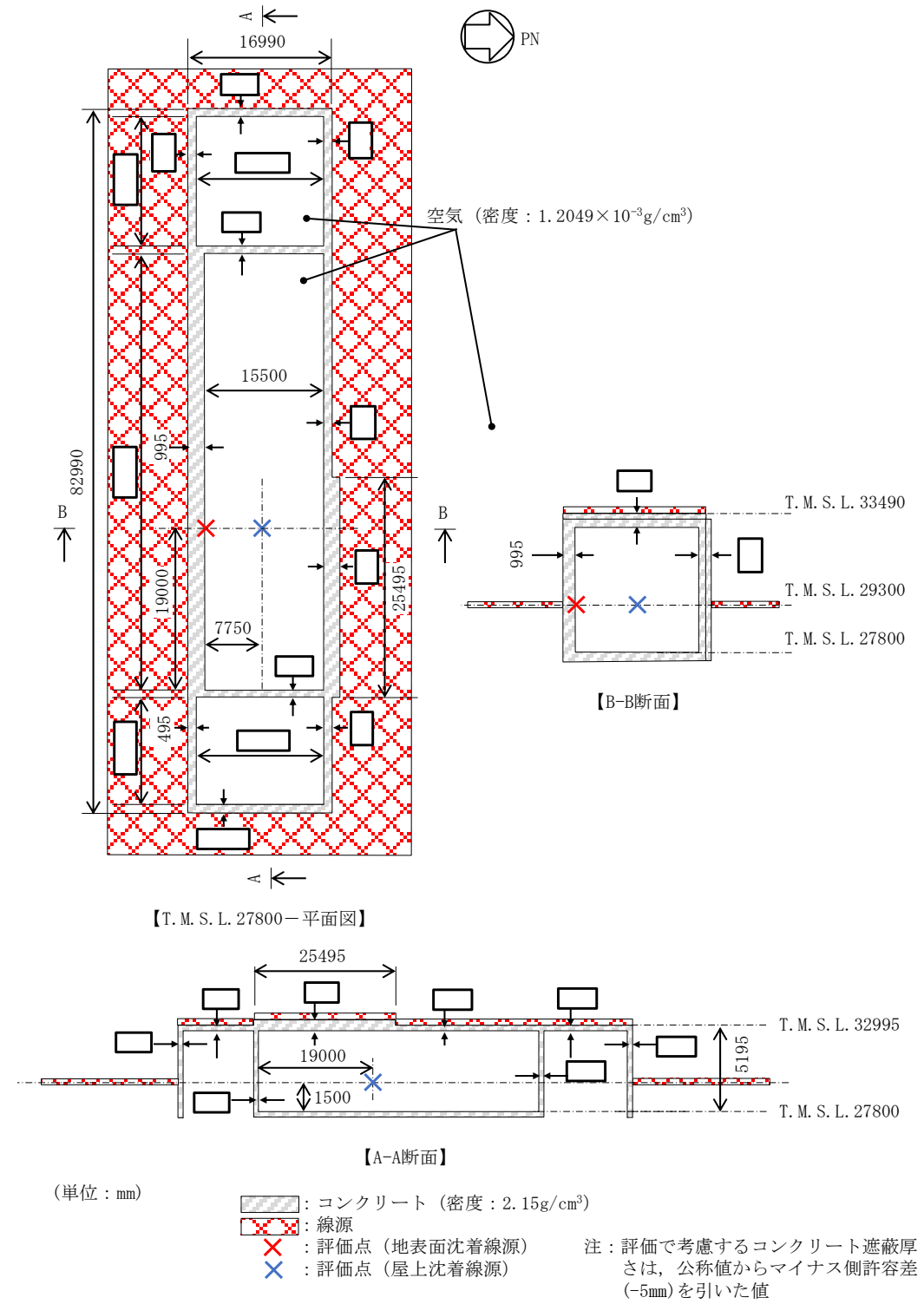
図4-9 グランドシャイン評価モデル (6/6) (緊急時対策所 (待機場所))
