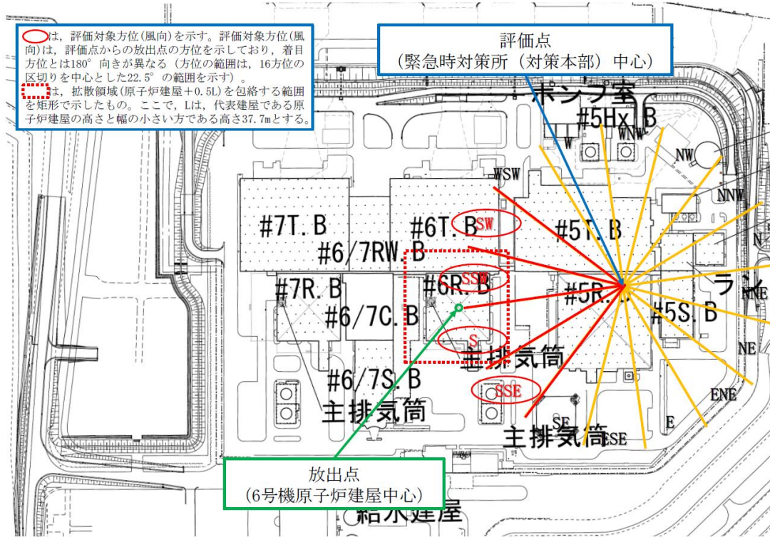
図4-3 評価対象とする風向 (1/4)
