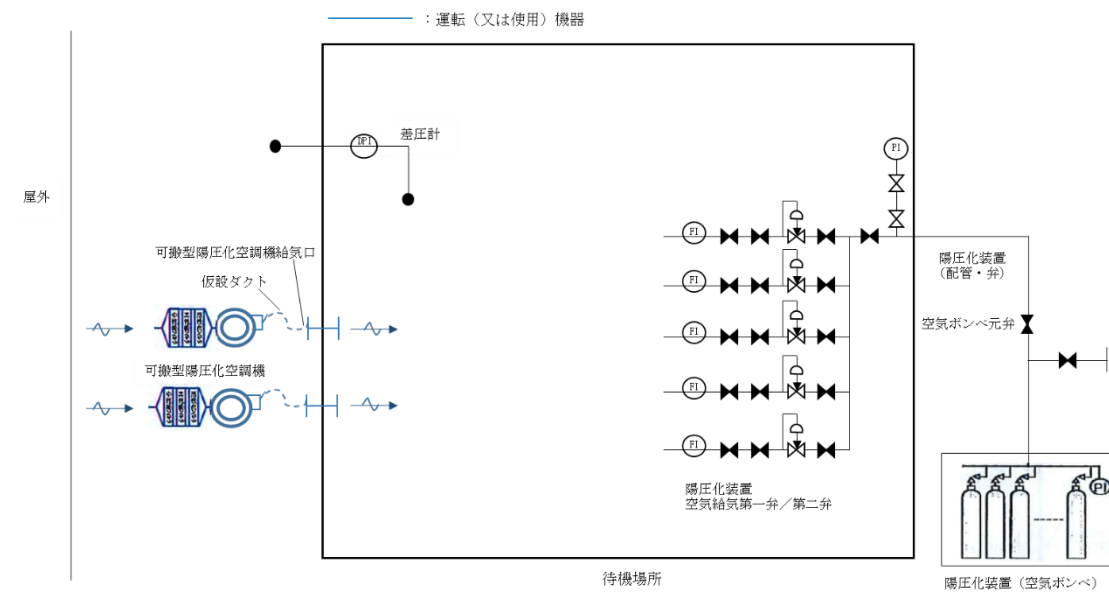
図3-6 緊急時対策所(待機場所)換気空調系構成図 (放射性雲通過前及び通過後:可搬型陽圧化空調機(待機場所)による陽圧化)
