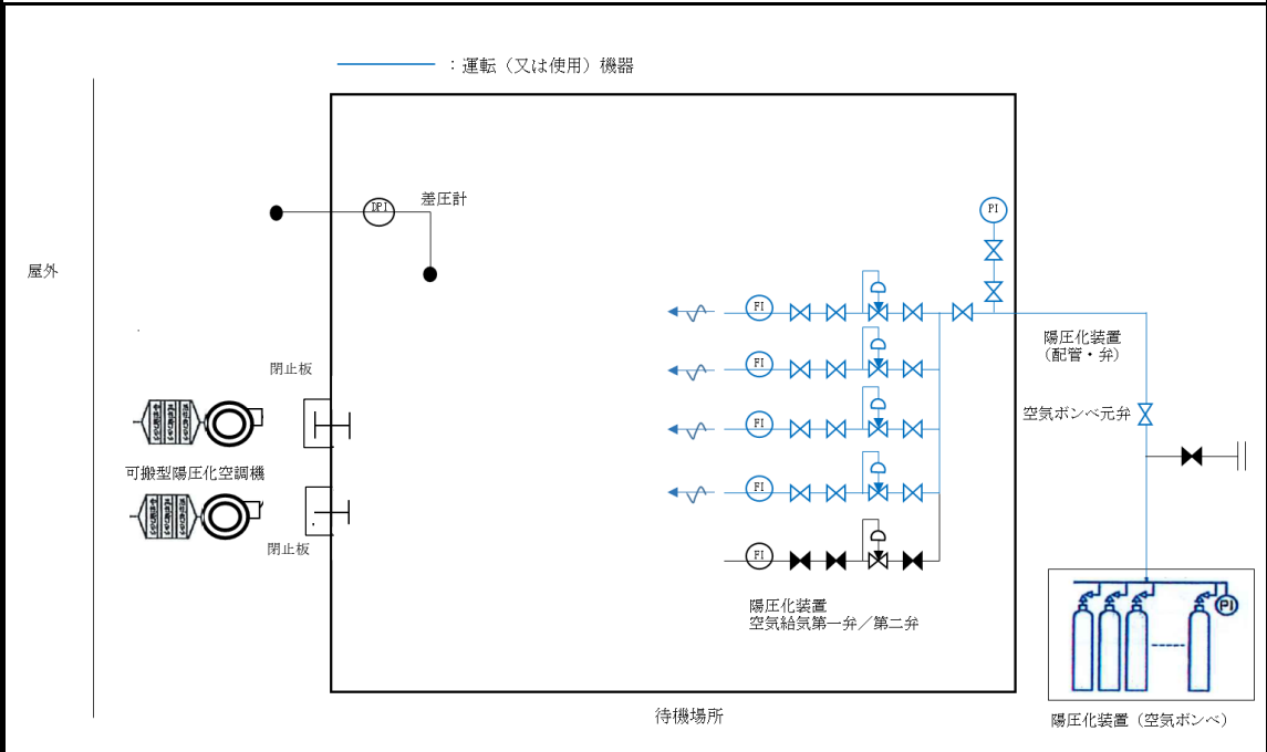
図3-7 緊急時対策所（待機場所）換気空調系 構成図 (放射性雲通過中：陽圧化装置（待機場所）による陽圧化)
