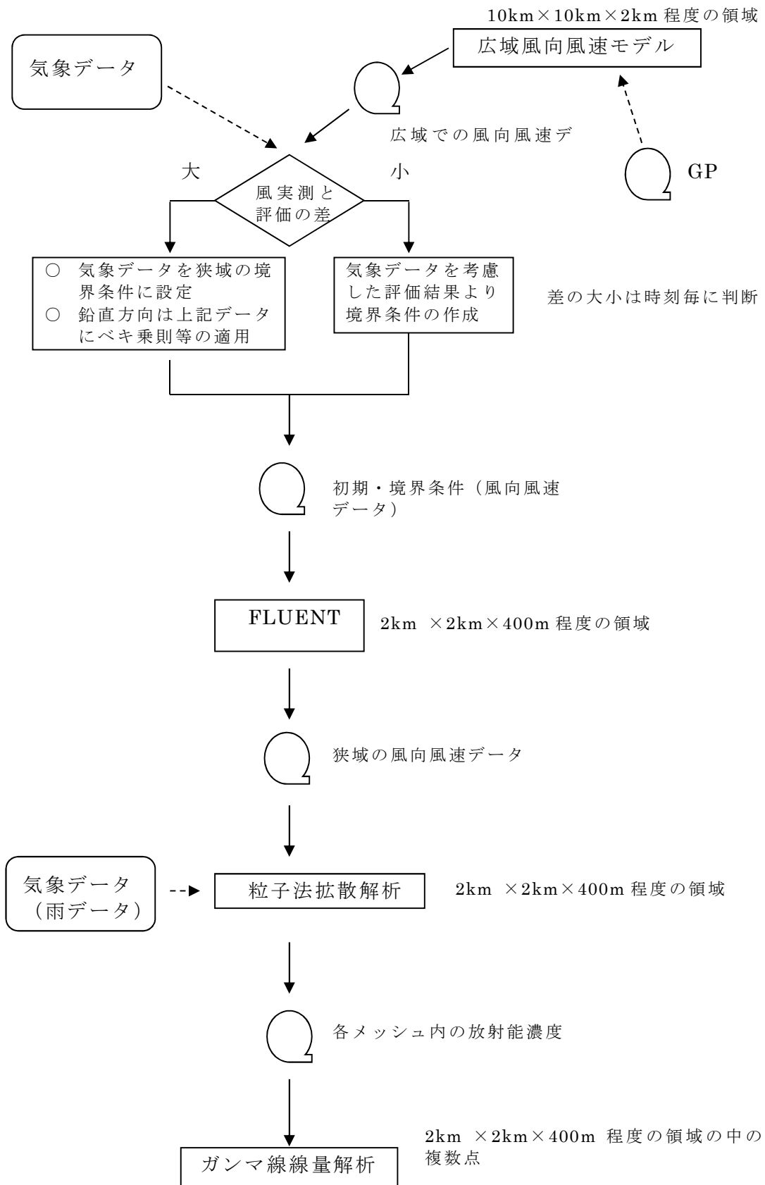
図 1 原子力発電所重大事故時空間線量評価システム（現行版）のフロー図
