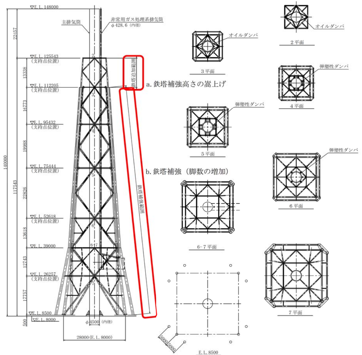
図 20 工事計画認可による耐震補強概要図【鉄塔部】
