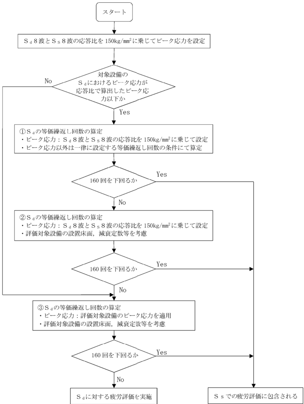
図3 弾性設計用地震動 S_e の等価繰返し回数の算出手順
