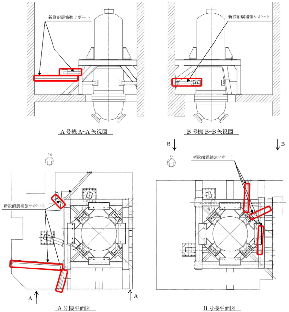
図 17 工事計画認可による耐震補強概要図
