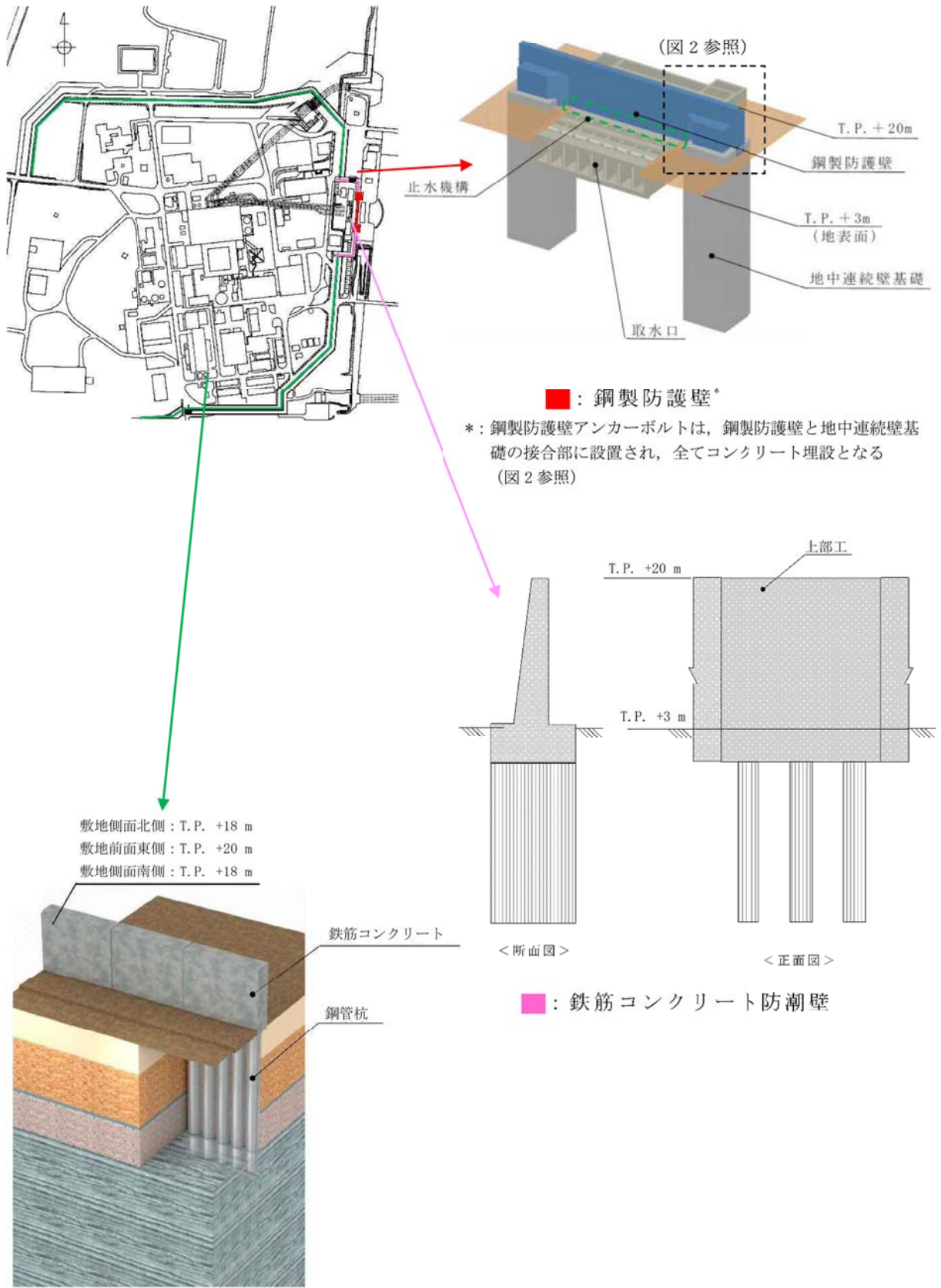
図1 東海第二 浸水防護施設の概要 (5/5)
