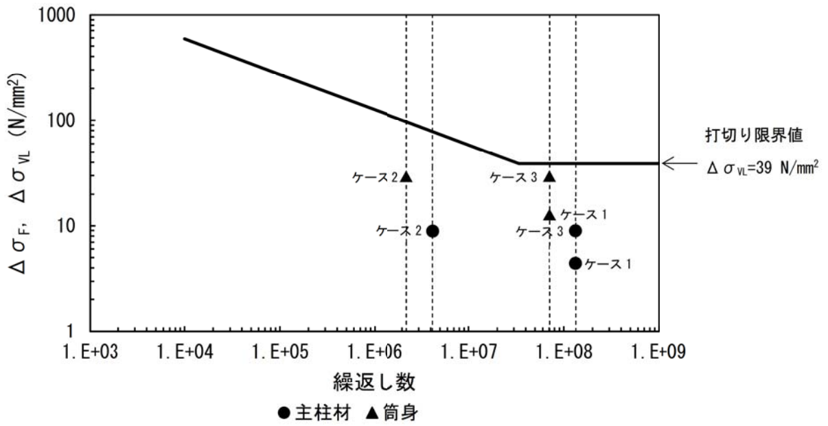
図-別紙 2-1 垂直応力範囲の繰返しによる疲労設計曲線
