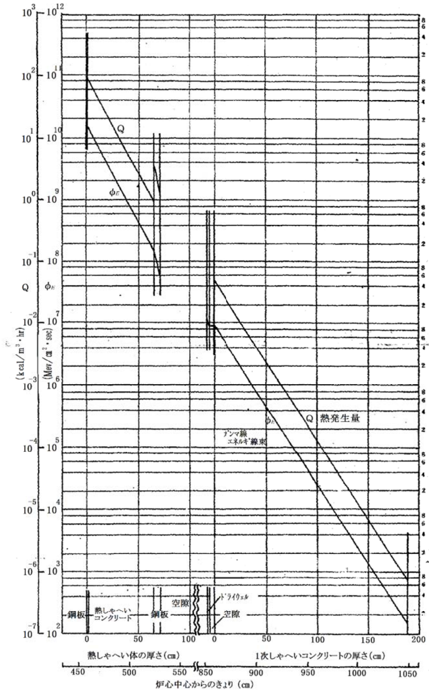
図-別紙-8-1 生体しゃへいコンクリート内におけるガンマ線束と発熱量分布
