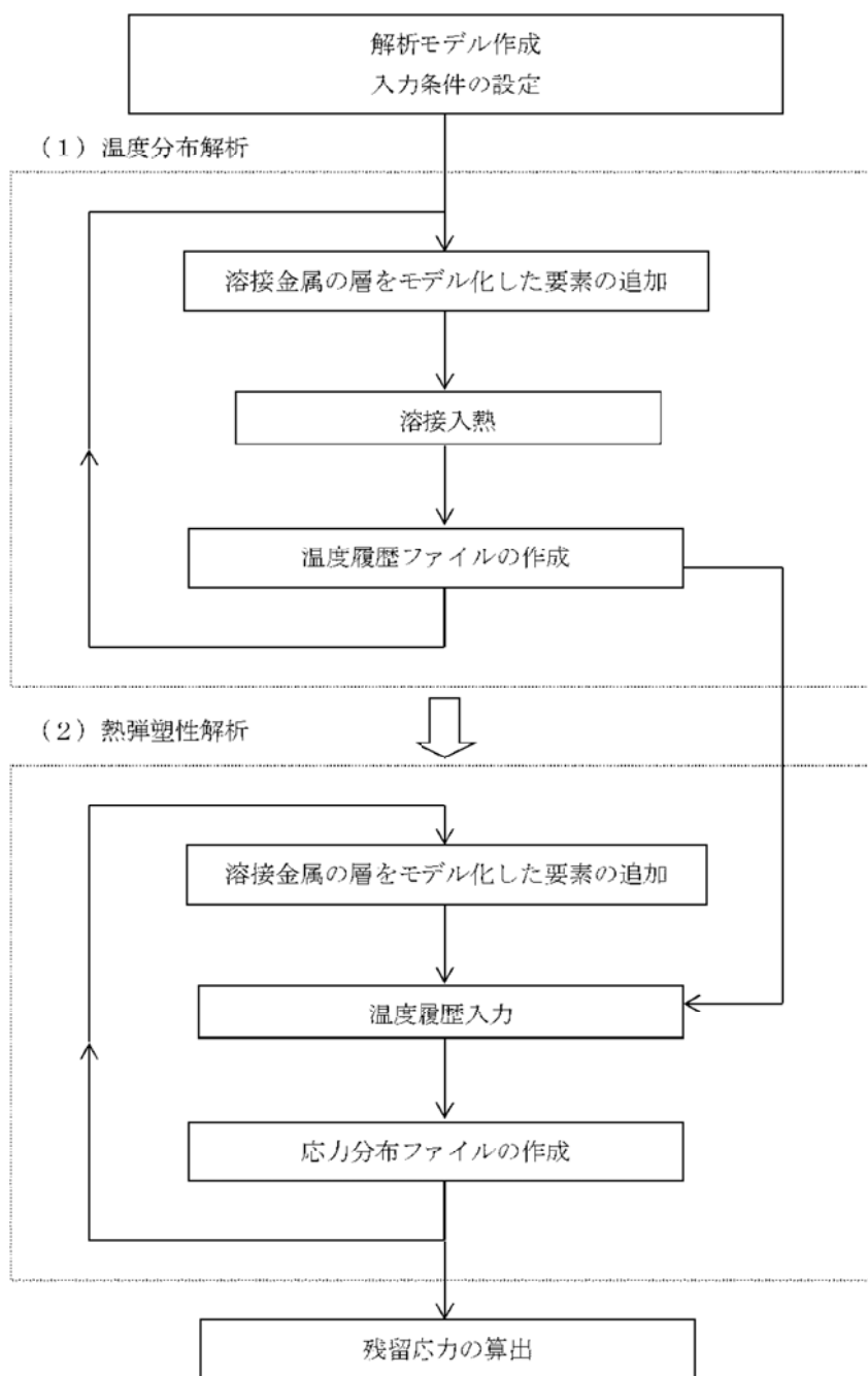
図2 溶接残留応力の解析手順
