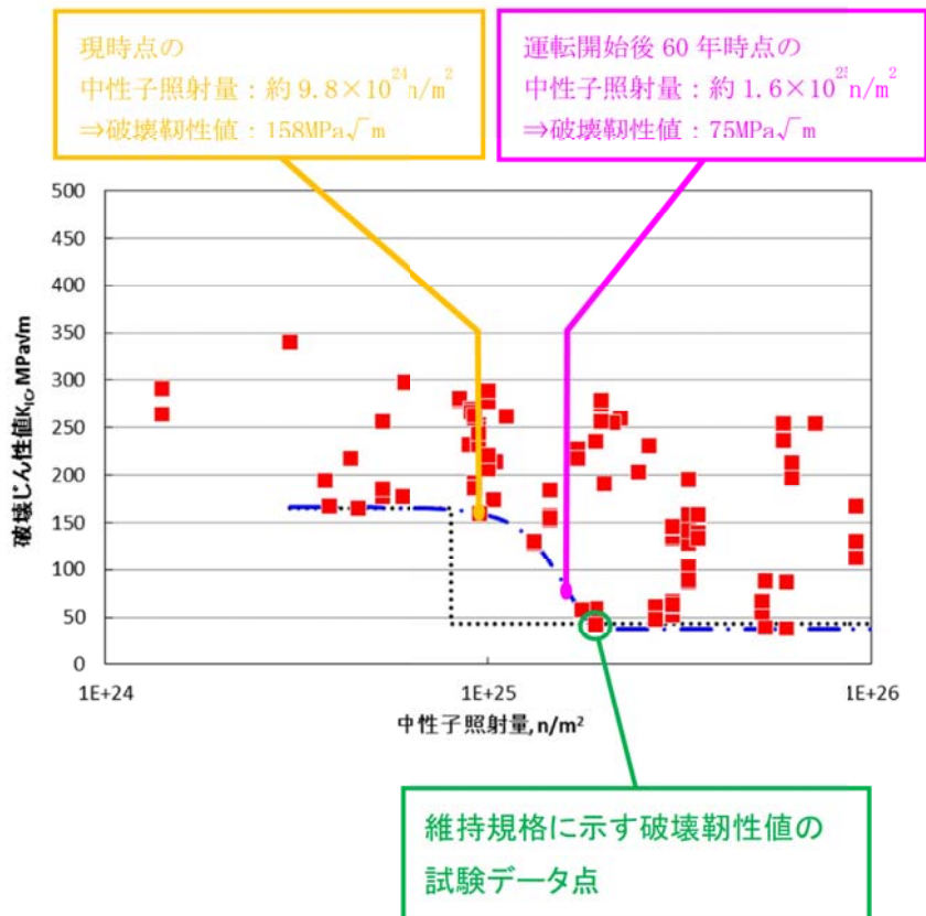
図3 破壊靱性評価式と試験データ
