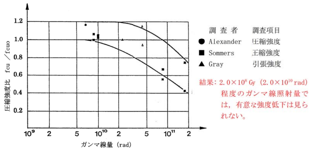
図4 ガンマ線照射したコンクリートの圧縮強度 (fcu) と照射しないコンクリートの圧縮強度 (fcuo) の比 2)
