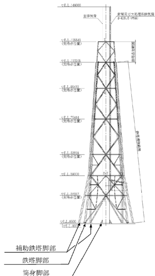
主排気筒 概要図
