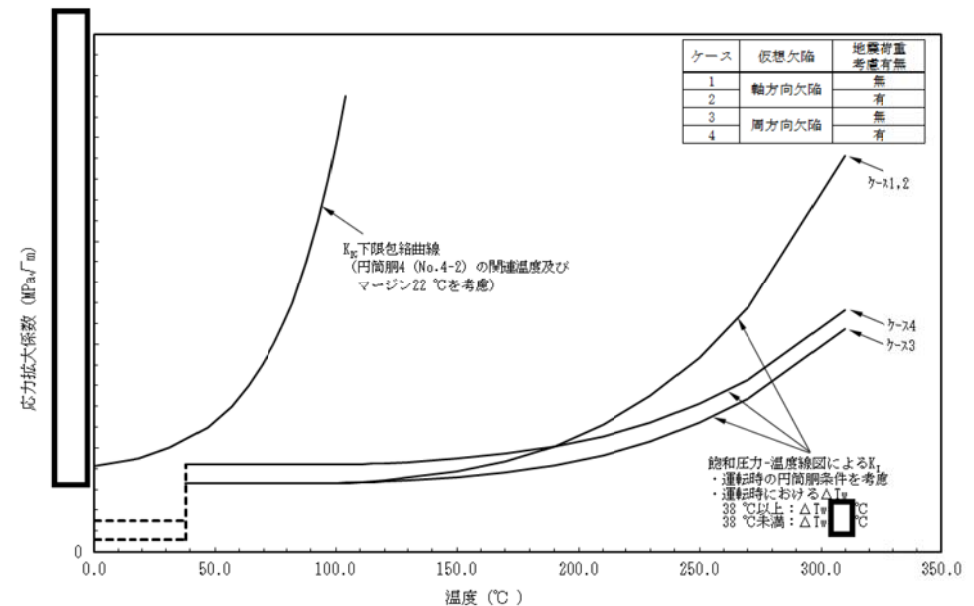
K_{IC} 下限包絡曲線と K_I 曲線(原子炉压力容器胴: 炉心臨界時)
