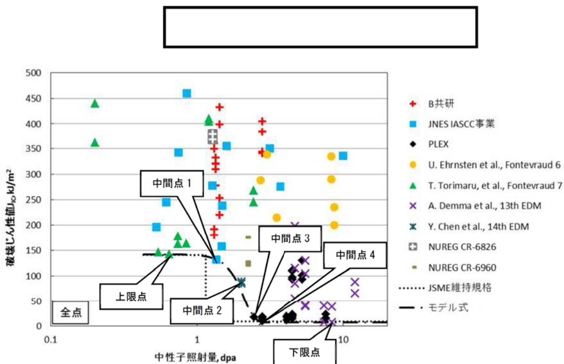
図 3-1 全点データを使用した破壊靱性評価式
