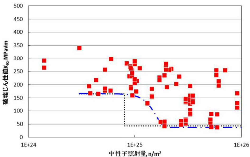
図 4-1 破壊靱性評価式
