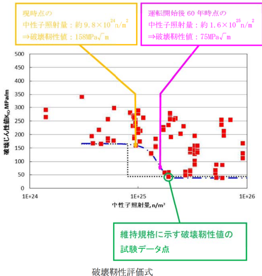
図7 破壊靱性評価式と試験データ
