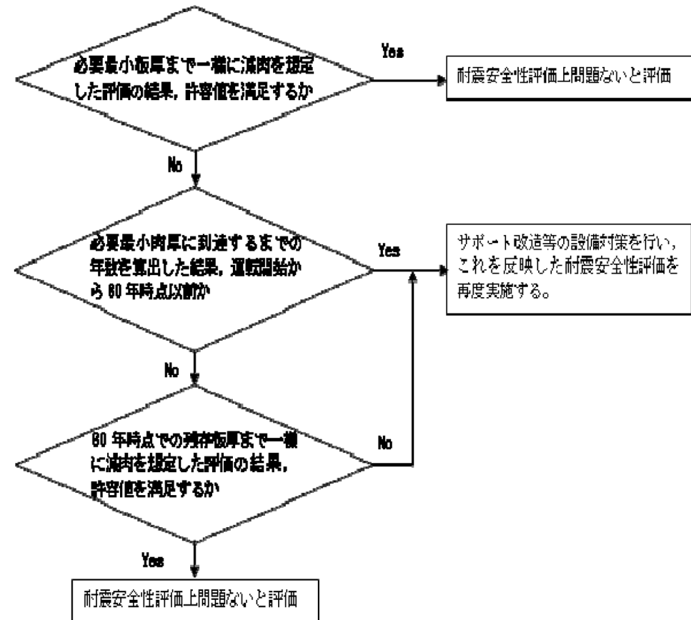
腐食(流れ加速型腐食)(配管)の耐震安全性評価フロー
