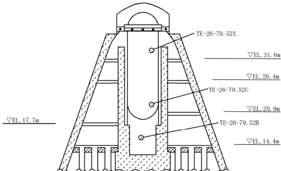
図-別紙 4-1 温度測定位置図
