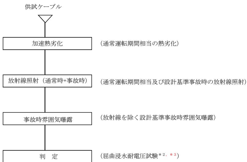
図 1.1 同軸ケーブル長期健全性試験手順（電気学会推奨案）
