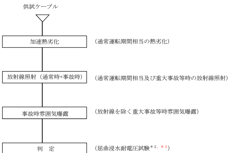
図 1.3 同軸ケーブル長期健全性試験手順（電気学会推奨案）
