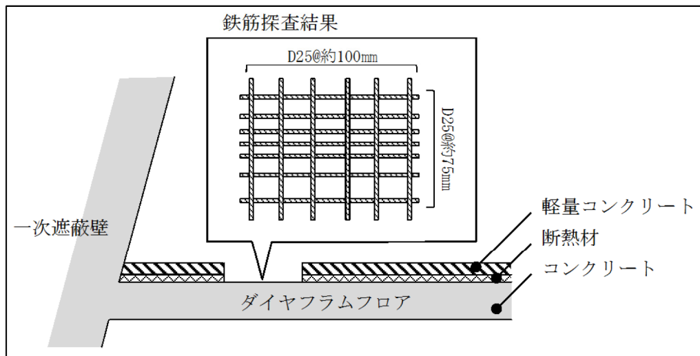
図 4. 1. 1-2 ダイアフラムフロア概要図
