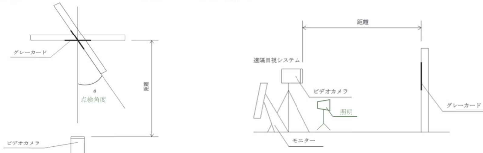
検証方法のイメージ図
