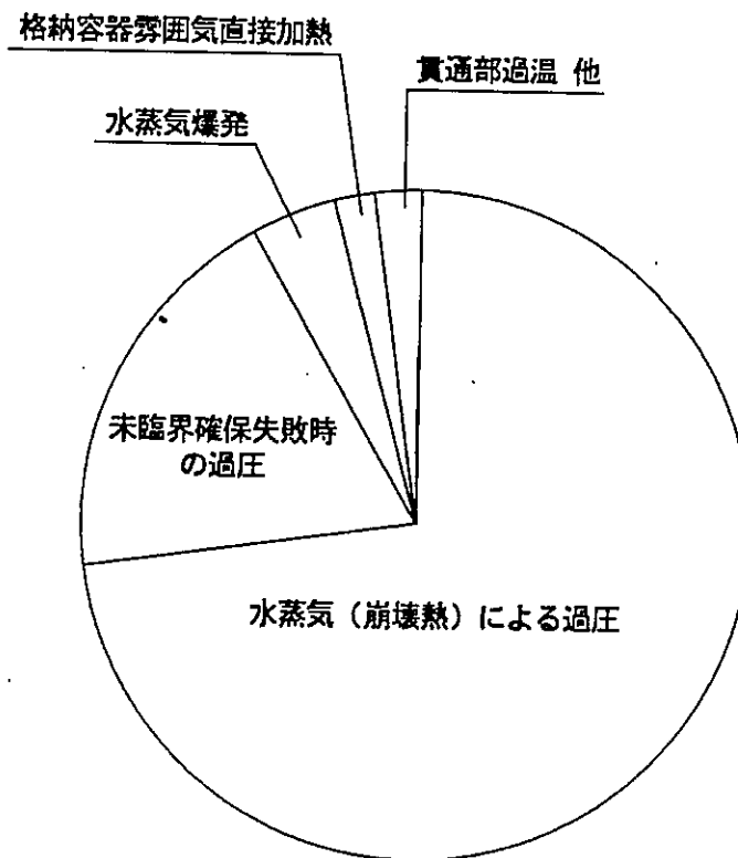
図-2 炉心の健全性に関するPSA結果
